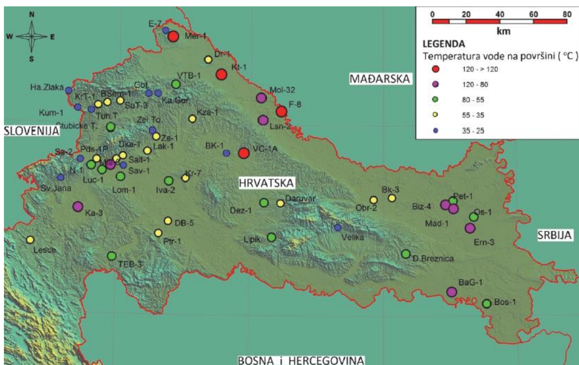
Slika 2-2. Prikaz bušotina geotermalnih polja (Kolbach i dr., 2018)
