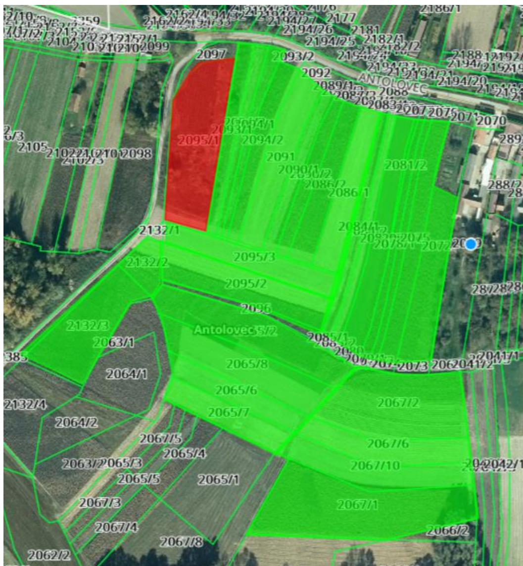
Slika 7-14. Prikaz potencijalnog rasporeda staklenika grijanih geotermalnom energijom direktnog sustava iskorištavanja (DGU, 2020)
