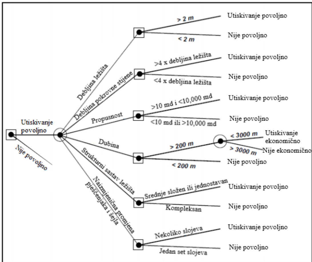
Slika 4-2. Stablo odlučivanja kao prvi dio opsežnog geološkog modela (Nadeem i dr., 2005)
