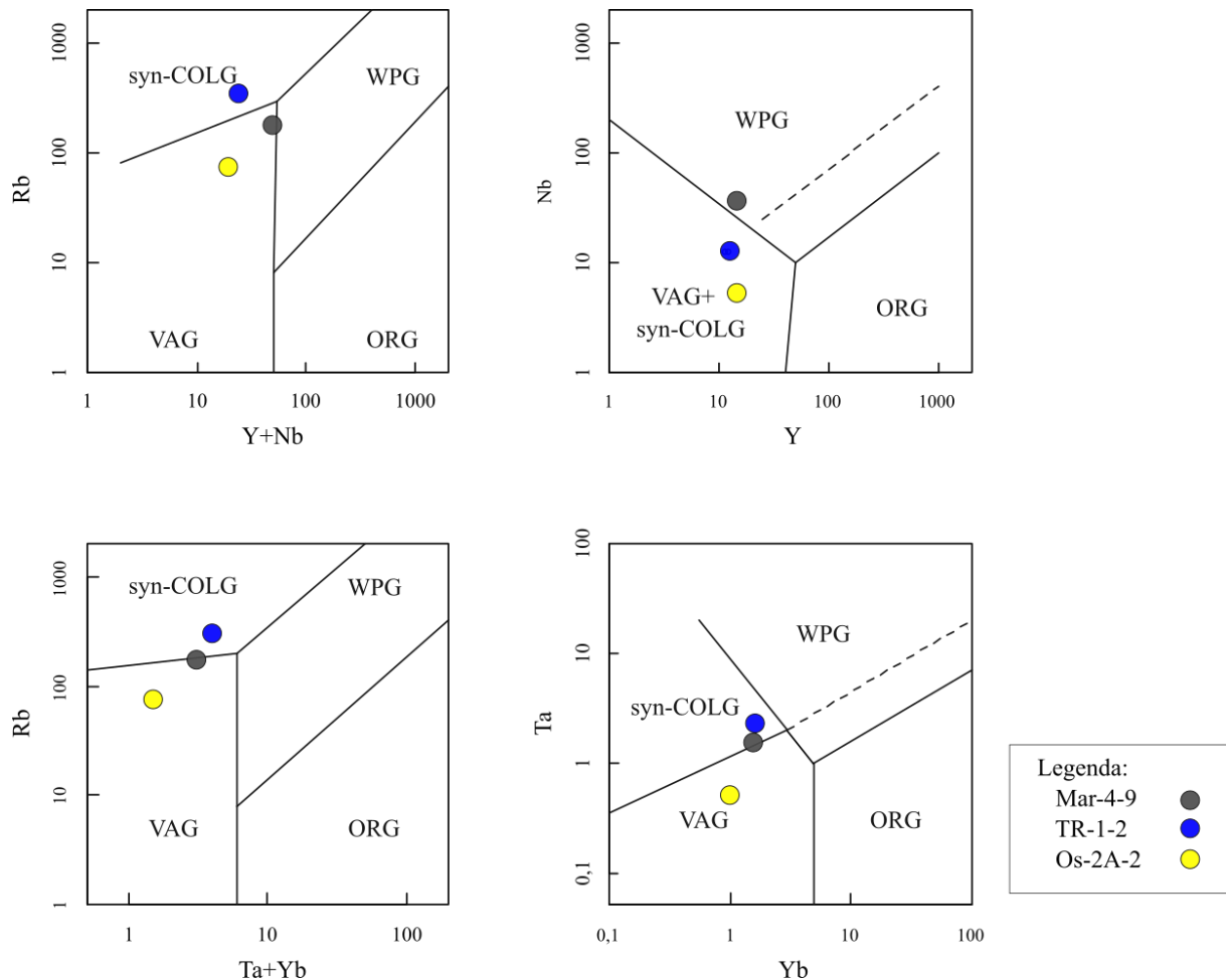
Slika 12.32 Diskriminacijski dijagrami za razlikovanje tektonskog porijekla granita (Pearce i dr., 1984) za analizirane stijene istočnog dijela Dravske depresije izuzevši područje Obod. WPG- graniti unutar ploče (eng. within plate granite ), syn-COLG sinkolizijski graniti (eng. syncollisional granite ), VAG-graniti vulkanskog luka (eng. volcanic arc granite ); ORG-graniti oceanskog hrpta (eng. ocean ridge granite ).
