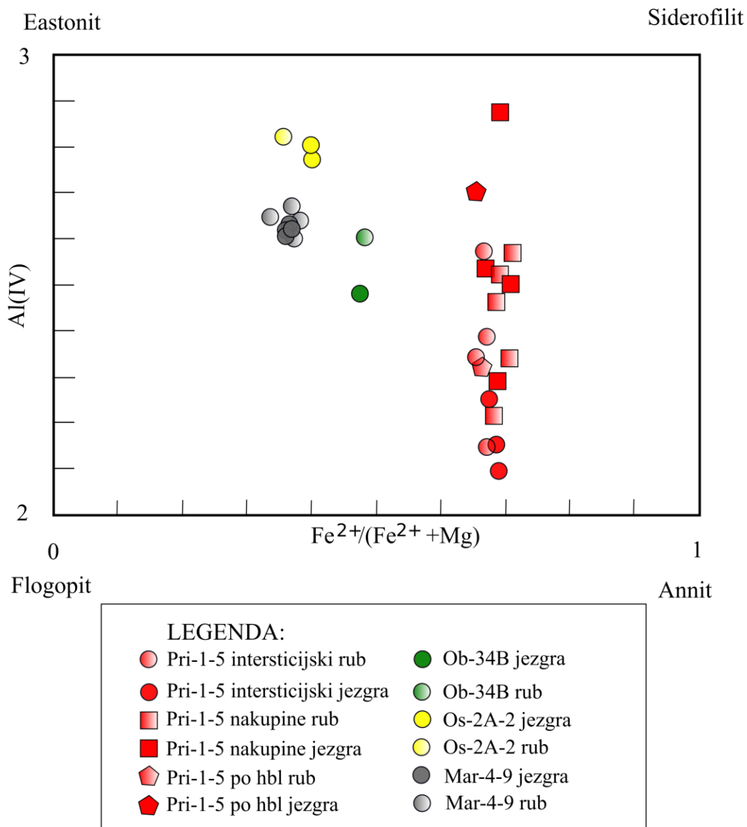
Slika 9.3 Klasifikacijski dijagram \text{Fe}^{2+}/(\text{Fe}^{2+}+\text{Mg})-\text{Al}(\text{IV}) analiziranog biotita.
