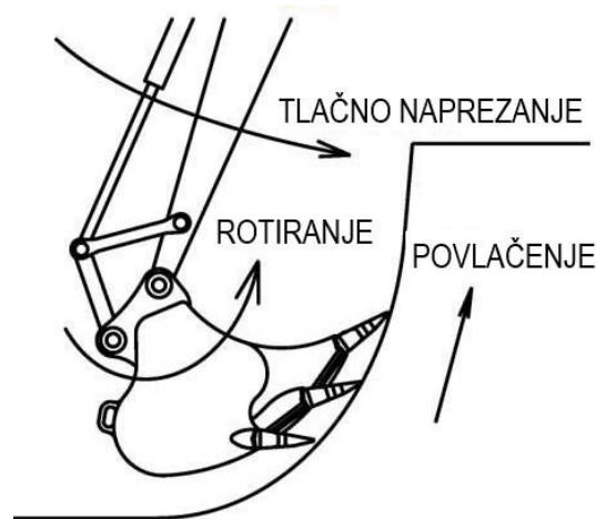
Slika 4.19. Dubinski način otkopavanja rijačem s više zubi na hidrauličnom bageru (www.digrock.com)
