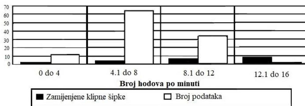
Slika 3-4. Odnos prosječnog broja zamijenjenih klipnih šipki u jednom remontu i broja hodova u minuti klipne sisaljke (Mottramu, 1991)
