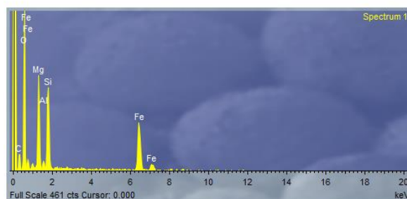
Slika 55. Energetsko disperzivni spektar zrna ortopirosena iz uzorka serpentinita oznake 205/11.
