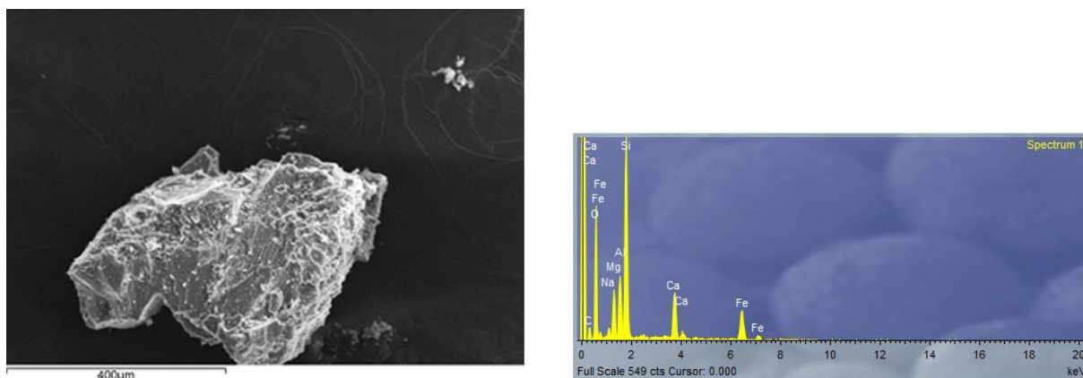
Slika 56. Energetsko disperzivni spektar zrna amfibola iz uzorka amfibolskog škriljavca oznake 205/1.
