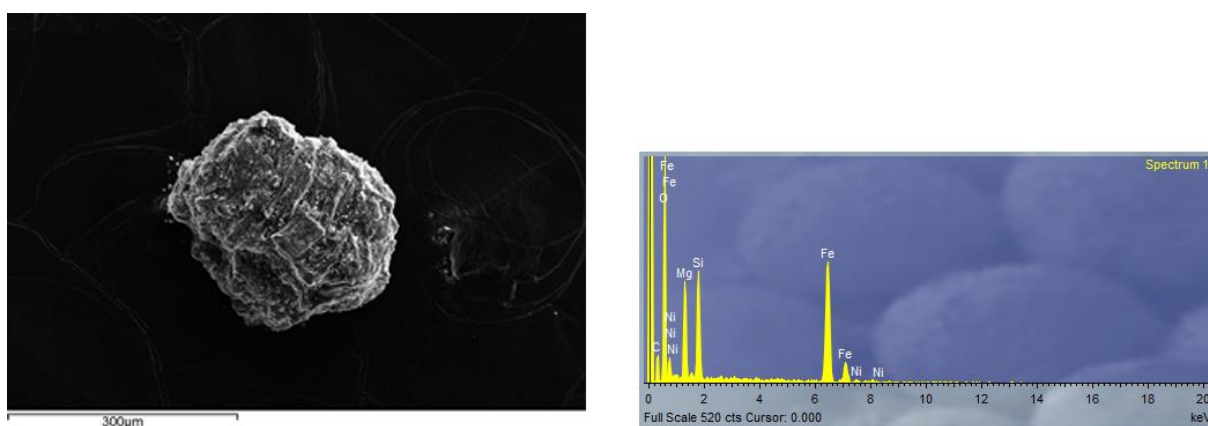
Slika 52. Energetsko disperzivni spektar zrna serpentina iz uzorka serpentinita oznake 205/11, u kojem je utvrđena i prisutnost Ni.
