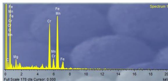
Slika 54. Energetsko disperzivni spektri zrna serpentina i kromita iz uzorka serpentinita oznake 205/11.
