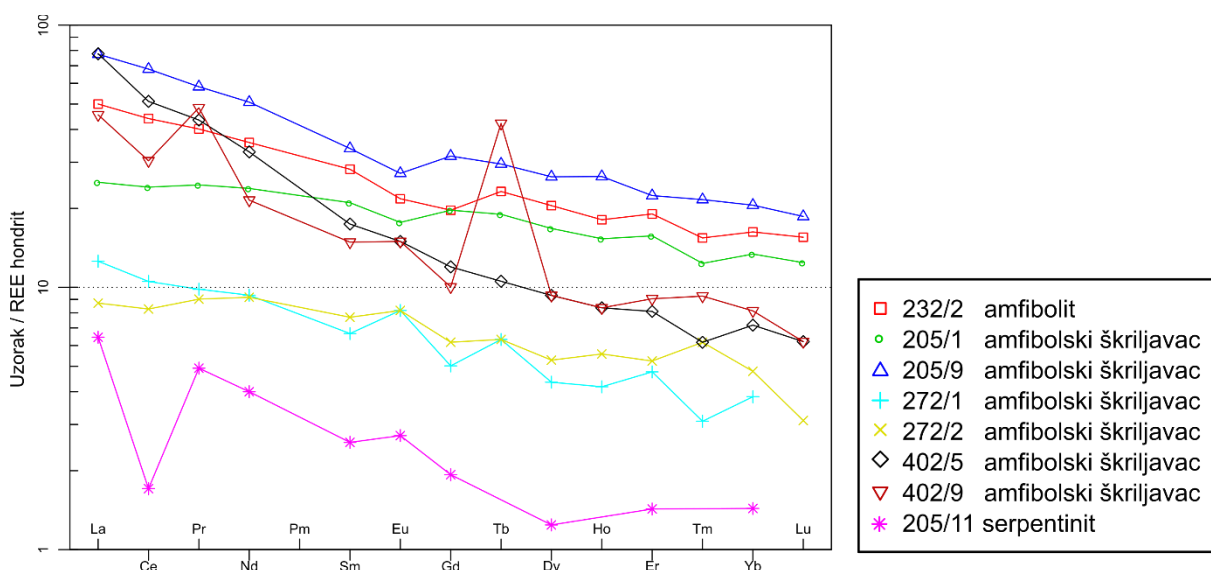
Slika 51. Obrazac raspodjele vrijednosti koncentracija elemenata rijetkih zemalja u uzorcima amfibolita, amfibolskog škrljavca i serpentinita, normaliziranih na hondrit prema Boynton (1984) .
