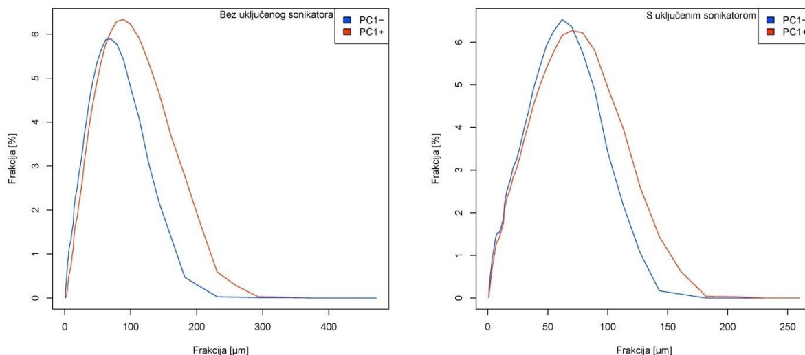
Slika 18. Krivulja odnosa veličine zrna i pripadajuće zastupljenosti za skupinu uzoraka PC1.
