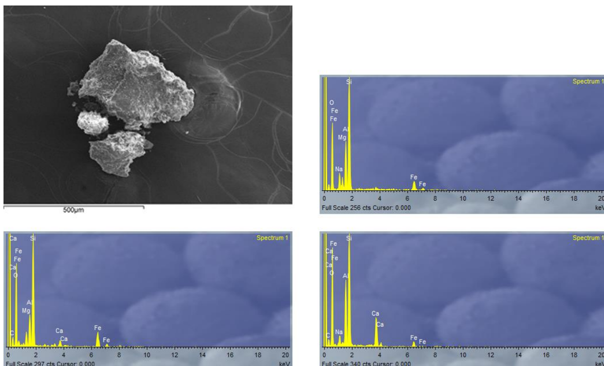
Slika 57. Energetsko disperzivni spektri zrna amfibola iz uzorka amfibolskog škriljavca oznake 232/2.
