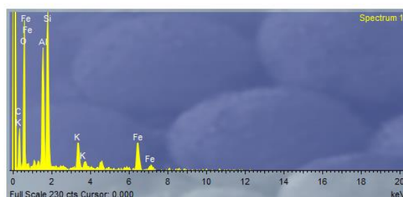
Slika 58. Energetsko disperzivni spektri zrna biotita iz uzorka amfibolskog škriljavca oznake 232/2.
