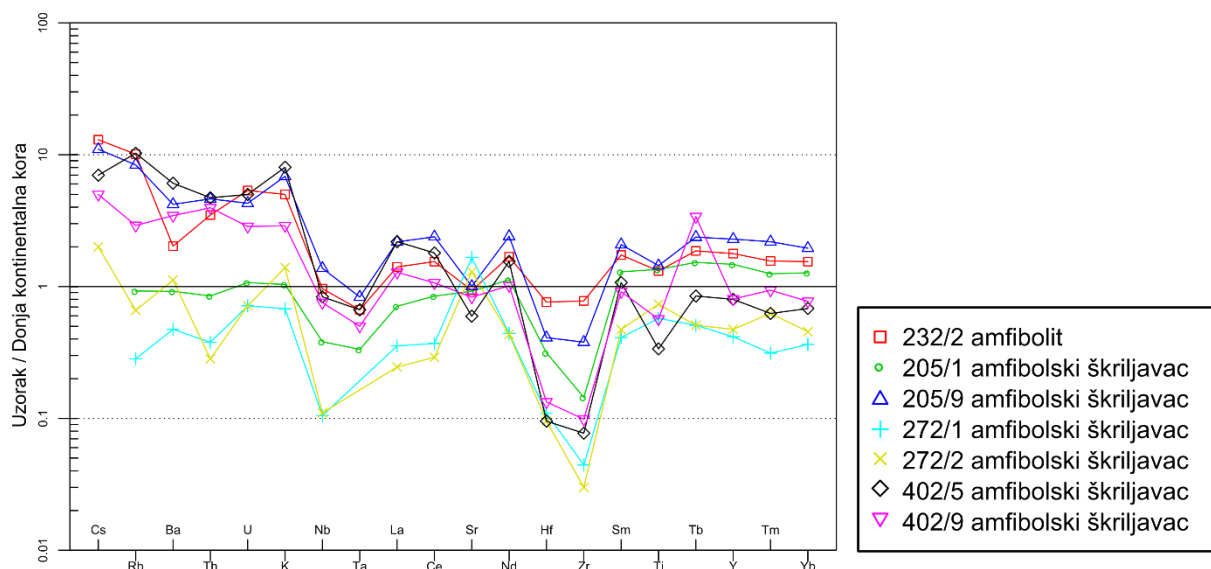
Slika 46. Obrazac raspodjele vrijednosti koncentracija nekompatibilnih elemenata u uzorcima amfibolita i amfibolskog škriljavca, normaliziranih na donju kontinentalnu koru prema Taylor i McLennan (1995) .
