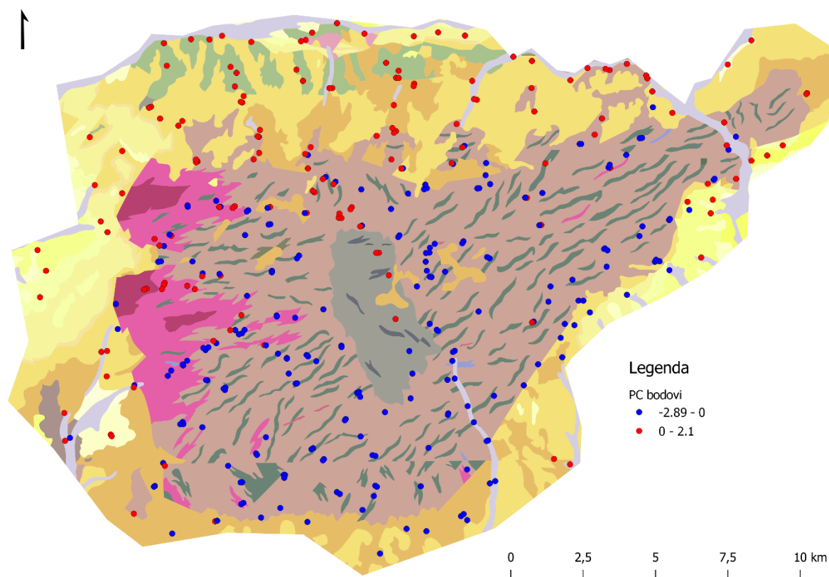
Slika 9. Prostorna raspodjela PC bodova dobivenih analizom glavnih komponentata na temelju koncentracija elemenata karakterističnih za stijene kiselijeg, odnosno bazičnijeg sastava. Geološka podloga i tumač oznaka kao na Sl. 4.
