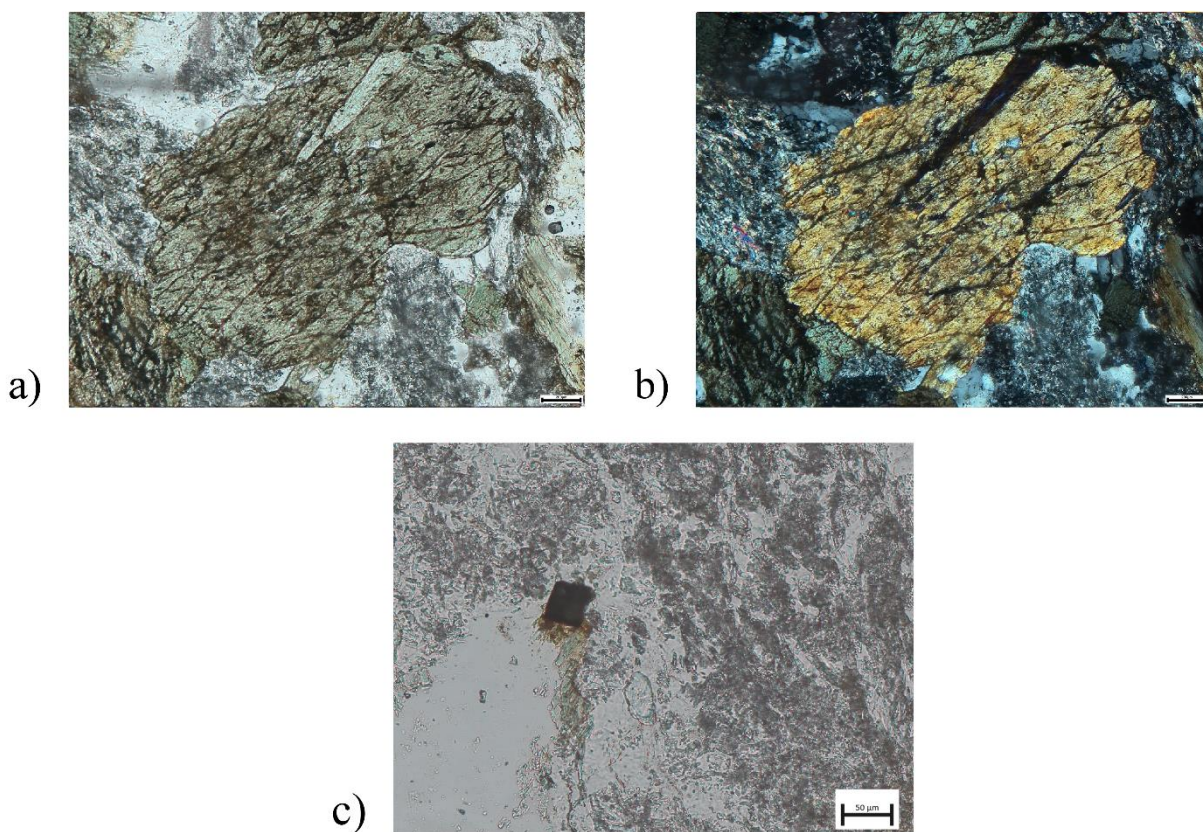
Slika 35. Uzorak PS 232/3 (a) bez analizatora, (b) s analizatorom i kvadratični presjek opâkog minerala.
