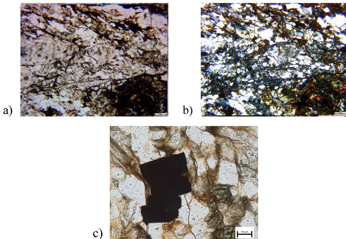
Slika 36. Uzorak PS 232/8 (a) bez analizatora, (b) s analizatorom i c) kvadratićni presjek opâkog minerala.
