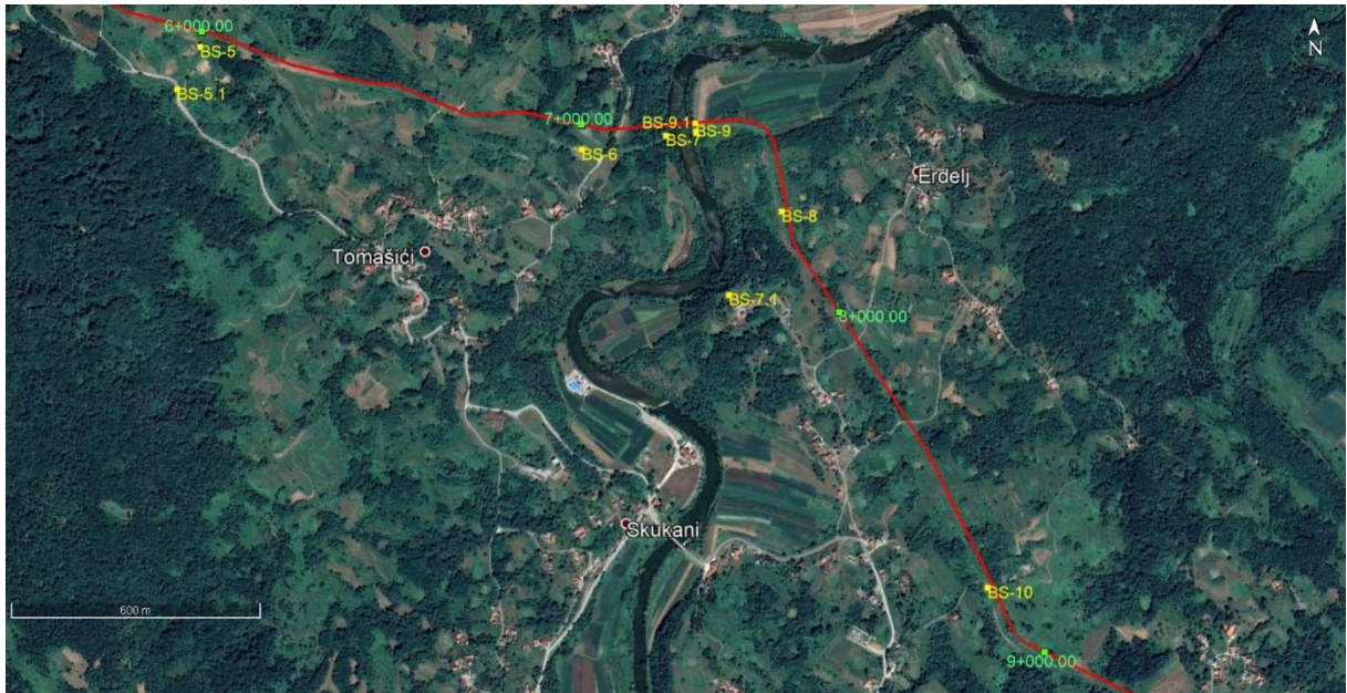
Slika 4-5 Pregledna karta područja trase magistralnog plinovoda Bosiljevo-Sisak DN 800/100 s ucrtanim terenskim točkama od stacionaže 6+000 do 9+000
