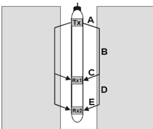
Slika 3-1. Sonda za zvučnu karotažu s jednim odašiljačem i dva prijemnika (Glover, 2012)
