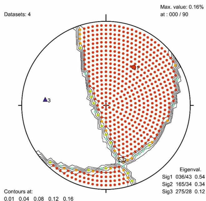
Slika 5.79. Strukturni dijagram pravih diedara za normalne rasjede strukturno-tektonske jedinice II (NR-2) s izračunom osi paleonaprezanja – najveća ( \sigma_1 ), srednja ( \sigma_2 ) i najmanja os paleonaprezanja ( \sigma_3 ).
