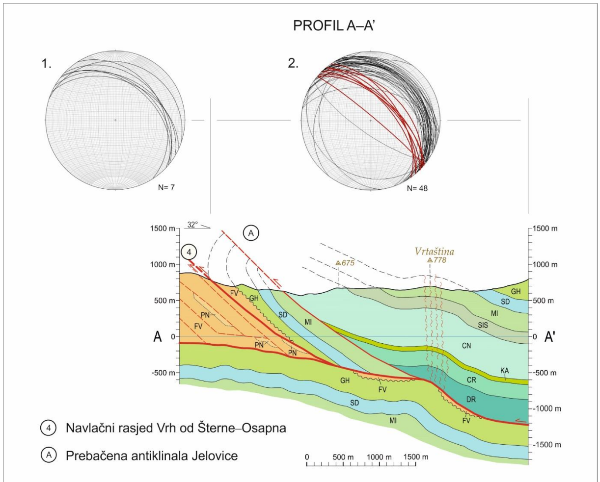
Slika 5.121. Geološki profil A–A'. Stereogram 1 – slojevitost u paleogenskim naslagama ljuskave strukture u podinskom krilu prebačene antiklinale Jelovice (oznaka A na profilu). Stereogram 2 – slojevitost naslaga u prebačenoj antiklinali Jelovice. Prebačena antiklinala Jelovice je vezana uz navlačni rasjed Vrh od Šterne–Osapna (oznaka 4 na profilu).
