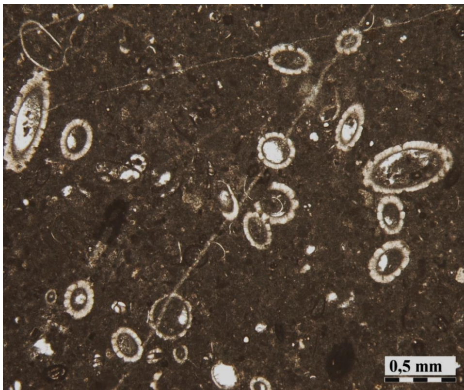
Slika 5.13. Mikrofajes algalnoga vekstona jedinice Kanfanar s brojnim presjecima vapnenačkih alga vrste Salpingoporella dinarica RADOIČIĆ; uzorak L-22 (45°28'5.7"N, 14°4'56.0"E).
