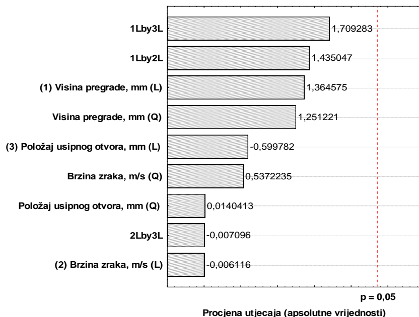
Grafikon 4 – 4 Procjena veličine utjecaja radnih parametara i njihovih međudjelovanja na maseno iskorištenje klase 2/1 mm – grupa „Z“
