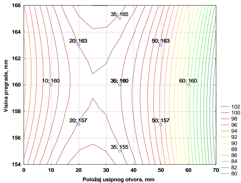
Slika 4 – 191 Nivo-linije regresijske plohe ovisnosti kvalitete koncentrata klase 2/1 mm o visini pregrade i položaju usipnog otvora – grupa „TP“
