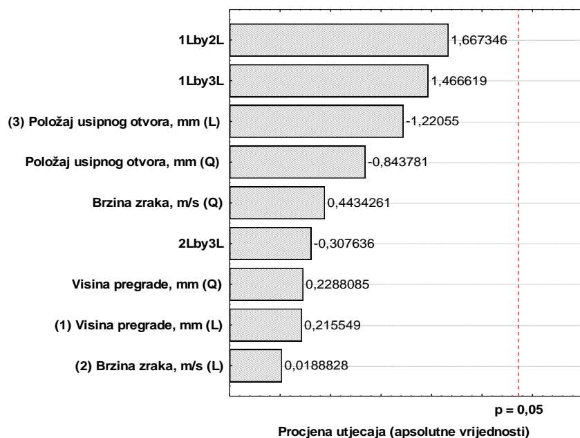
Grafikon 4 – 3 Procjena veličine utjecaja radnih parametara i njihovih međudjelovanja na kvalitetu koncentrata klase 2/1 mm – grupa „Z“
