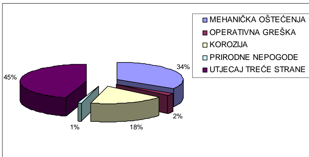
Slika 4-5. Podaci o uzrocima propuštanja naftovoda koje obuhvaća baza CONCAWE u postocima u razdoblju 2006. - 2010. godine, (CONCAWE, 2011).
