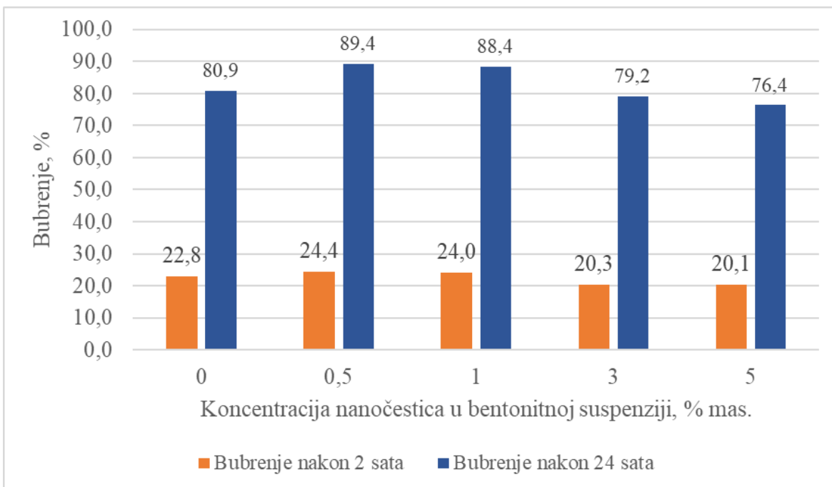
Slika 6-38. Bubrenje peleta u bentonitnoj suspenziji bez i s nanočesticama Al_2O_3 -20 nm izraženo u postocima nakon 2 i 24 sata
