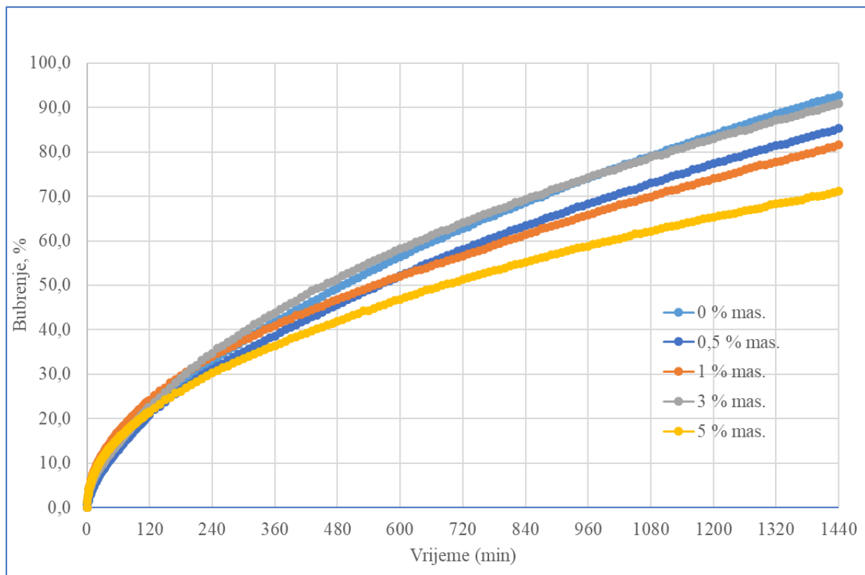
Slika 6-55. Bubrenje peleta u vodi i vodenoj suspenziji nanočestica Fe 2 O 3 -20 do 30 nm tijekom 1 440 minuta
