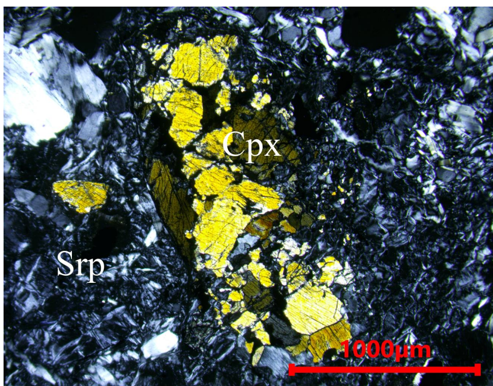
Slika 5.31. Nakupine klinopiroksena u uzorku spinelskog lhercolita Lj-2, a koje su najvjerojatnije posljedica djelomične rekristalizacije nekadašnjeg većeg zrna klinopiroksena. Cpx – klinopiroksen, Srp - serpentin, (N+).
