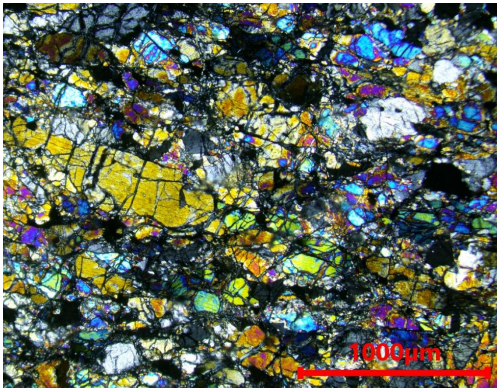
Slika 5.48. Ekvigranularna tabularna struktura u spinelskom leucitu 18Gv-4, (N+).
