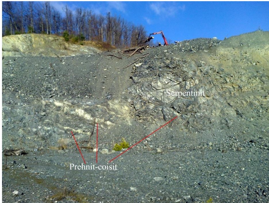
Slika 5.19. Zmijolika tijela bogata s prehnitom i coisitom u ritmičnoj izmjeni sa serpentinitom. Lokalitet Slatina.
