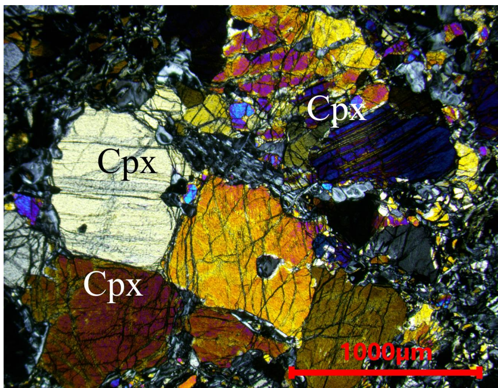
Slika 5.30. Nakupine klinopiroksena u spinelskom lhercolitu Zub-4. Opx – ortopiroksen, Cpx – klinopiroksen, (N+).
