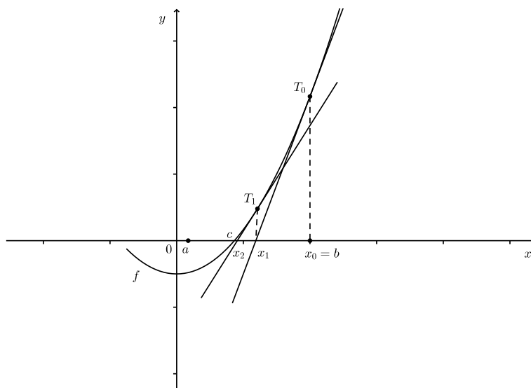
Slika 2: Newtonova metoda
