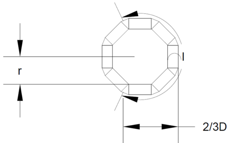
Slika 10-6 Poprečni presjek ciglenog dimnjaka sa zalomom 2/3 opsega
