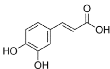
Kofeinska kiselina
