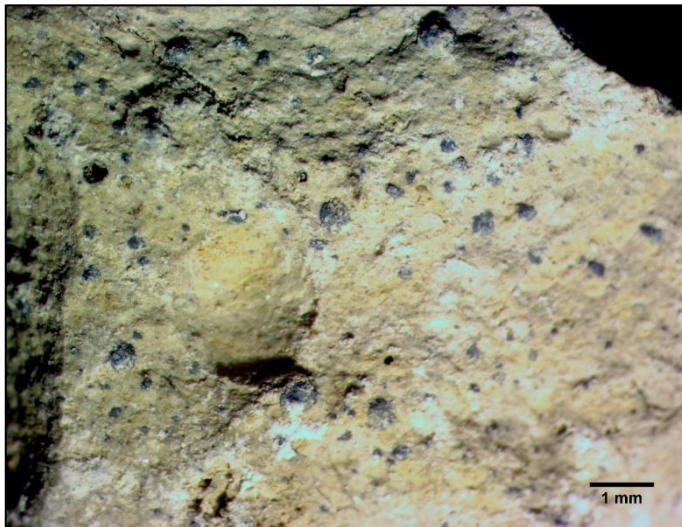
Slika 8 - 15 Fotografija uzorka boksita 6959.
