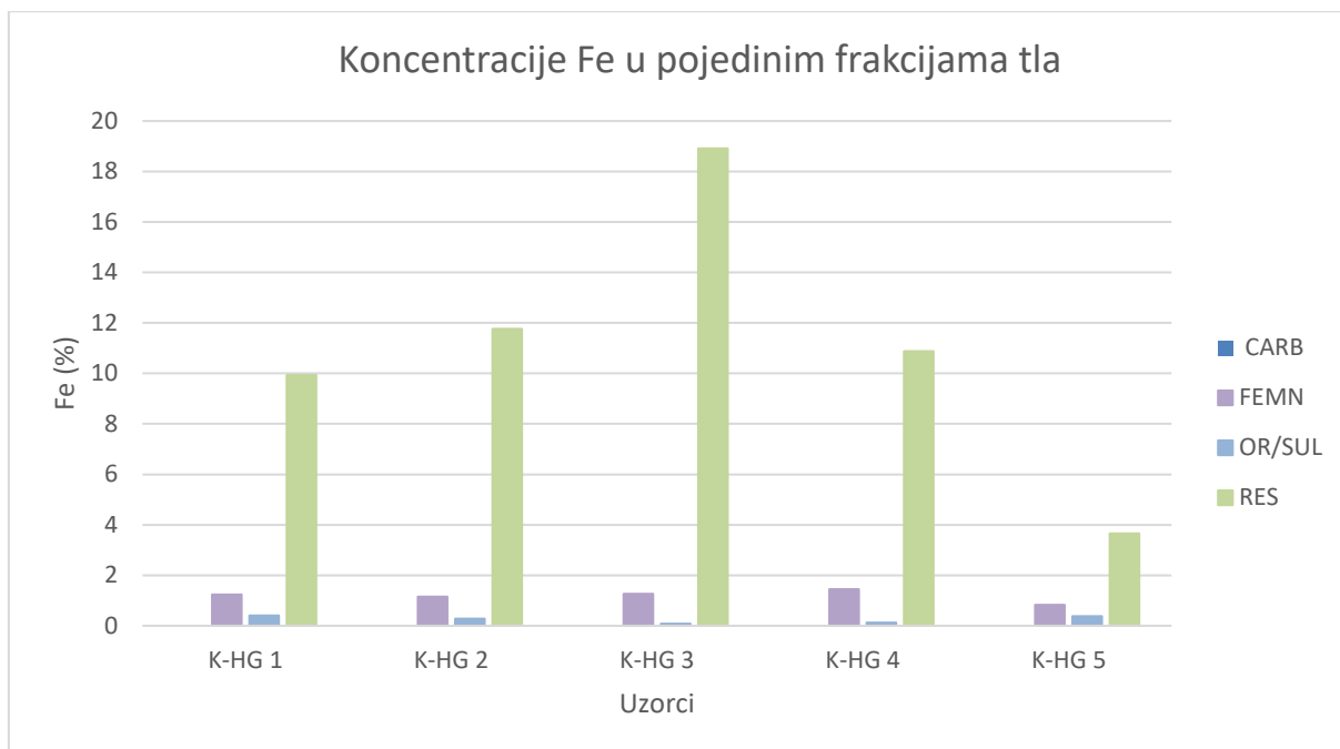
Slika 7–7. Koncentracije Fe(%) u pojedinim frakcijama tla.
