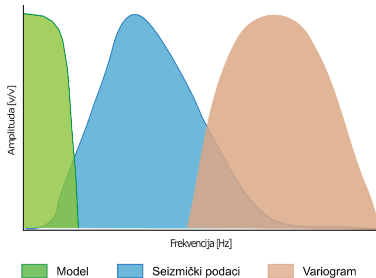
Slika 10-9 Frekvencijski spektri ulaznih podataka stohastičke inverzije
