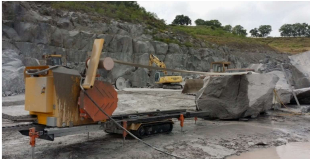
Slika 3-14: Dijamantna žična pila S800T (Promidžbeni materijal tvrtke Dazzini Machine, 2010.)
