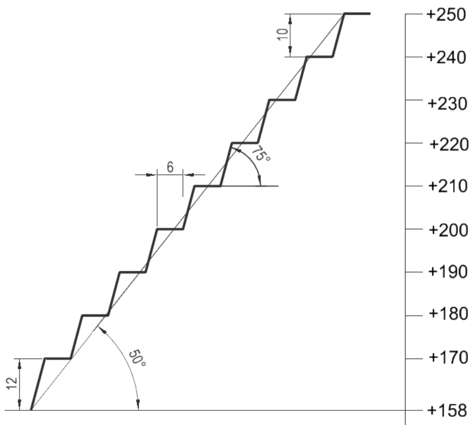
Slika 2-4 Presjek završe kosine zapadnog dijela Bukove Glave
