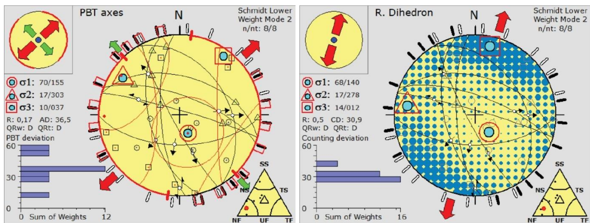
Slika 5.4 Prikaz proračunatih vektora glavnih osi naprezanja za prvu skupinu normalnih rasjeda. Na slici lijevo nalazi se sintetski žarišni mehanizam kojem su PBT metodom proračunate glavne osi paleonaprezanja. Na slici desno nalazi se beach-ball dijagram proračunat R. Dihedron metodom
