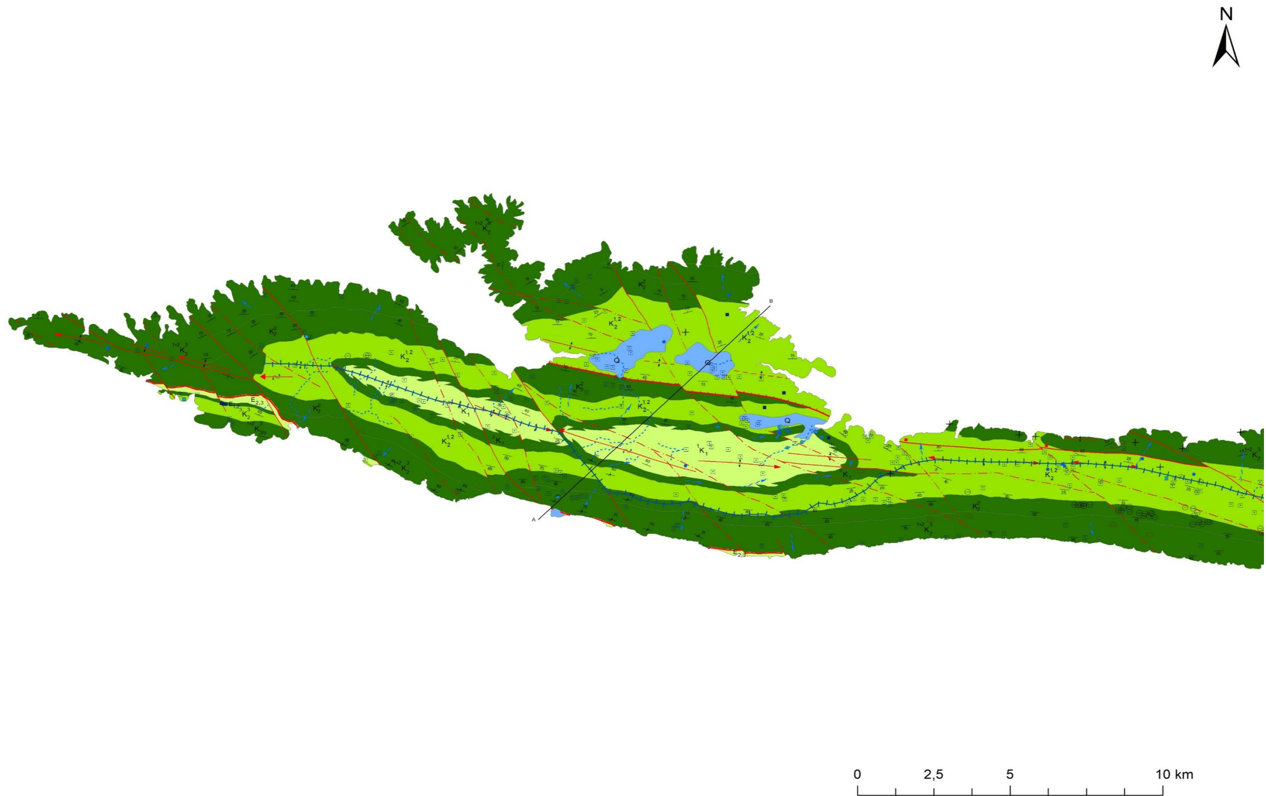
Slika 3-3. Hidrogeološka karta zapadnog i središnjeg dijela otoka Hvara
