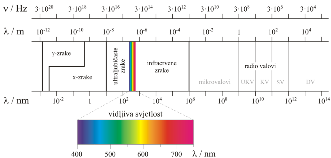
Slika 4-5. Spektar elektromagnetnog zračenja (Glossary, 2022)
