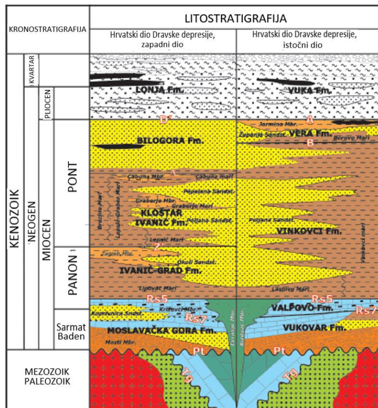
Slika 3.3. Formacije unutar hrvatskog dijela Dravske depresije (Malvić & Cvetković, 2013)
