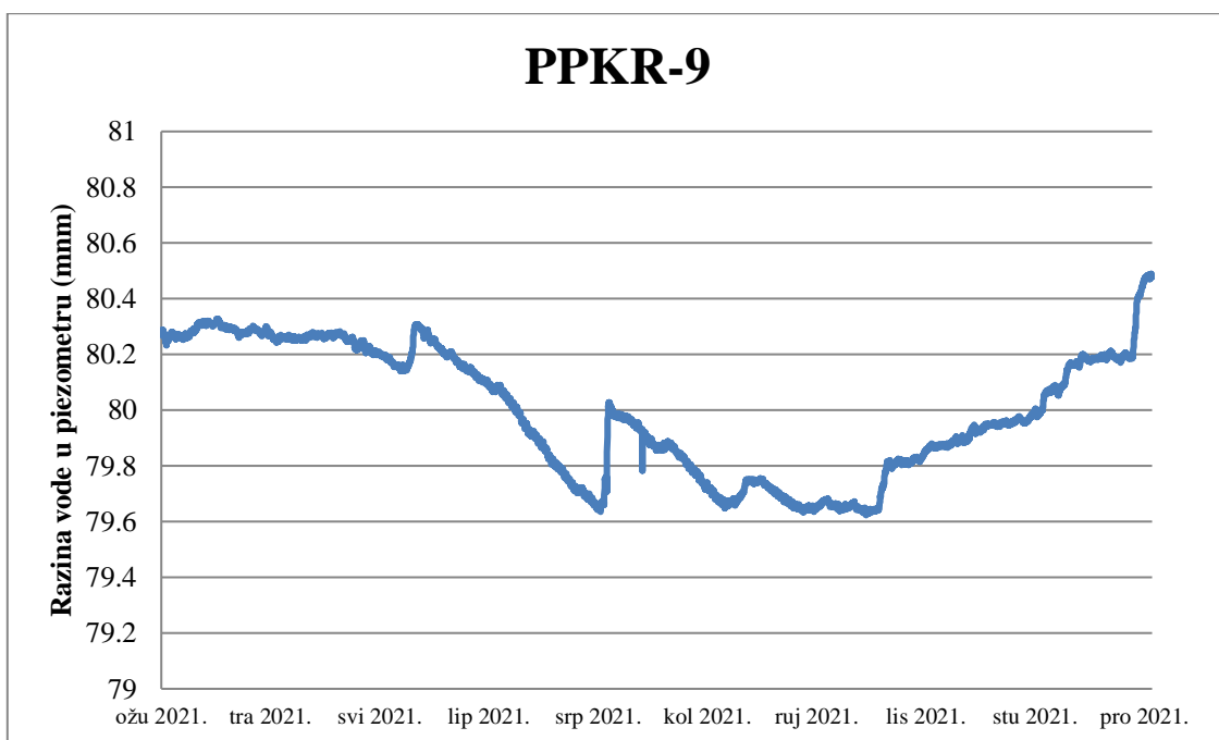
Slika 5.9. Korigirana razina u piezometru PPKR-9
