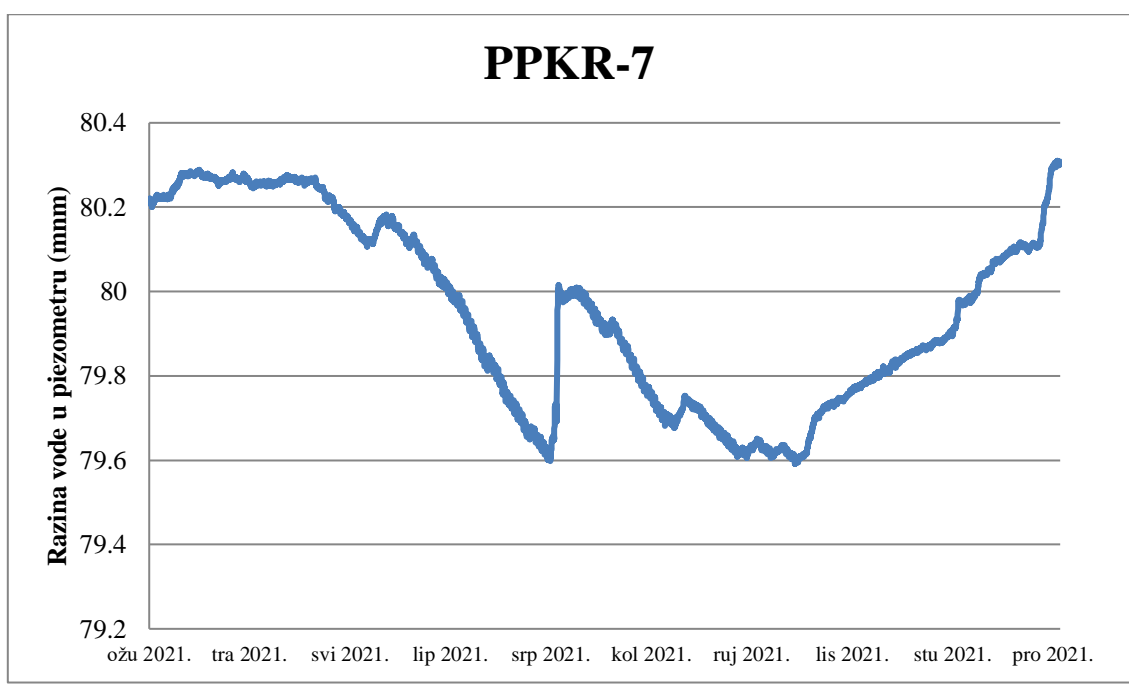
Slika 5.7. Korigirana razina u piezometru PPKR-7
