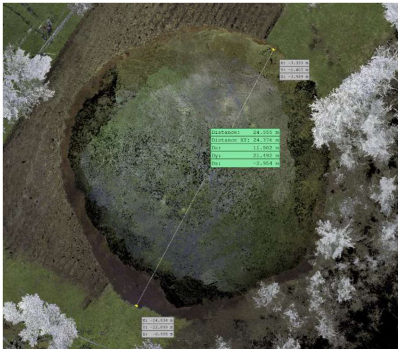
Slika 4-4. LiDAR-ska snimka najveće vrtače u Mečenčanima, promjer vrha vrtače (Tomac i dr., 2021)
