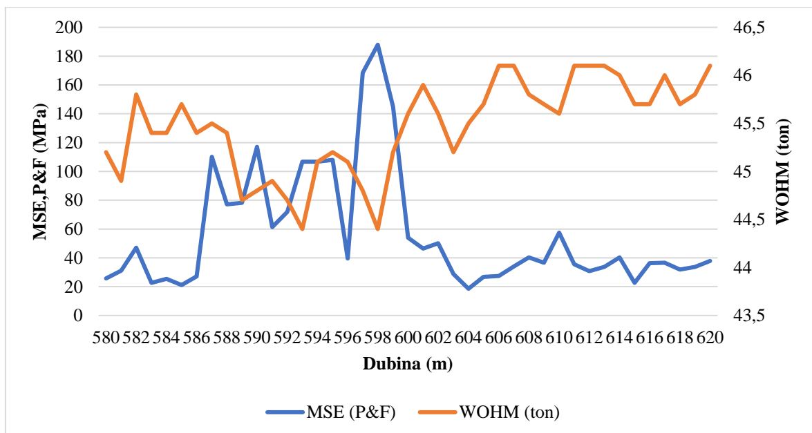
Slika 5-5. Promjena vrijednosti MSE i opterećenja na dlijeto – WOHM s promjenom dubine prema P&F modelu
