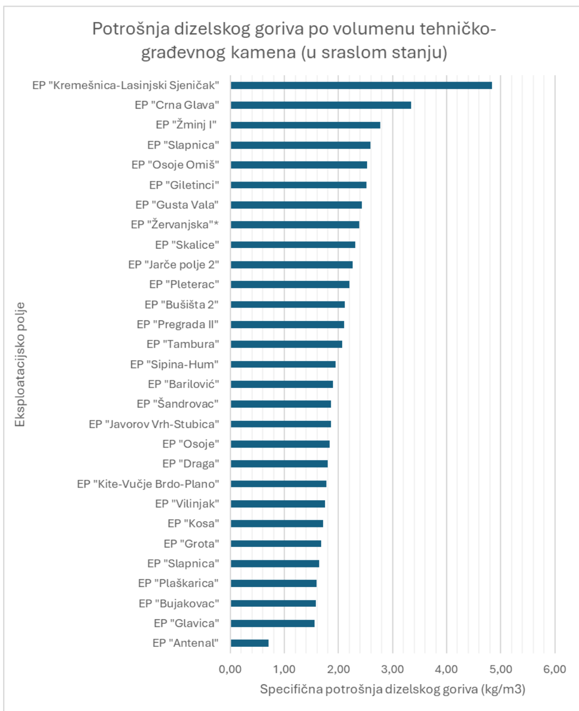
Slika 5-1. Rangiranje eksploatacijskih polja na temelju specifiĉne potrošnje dizelskog goriva
