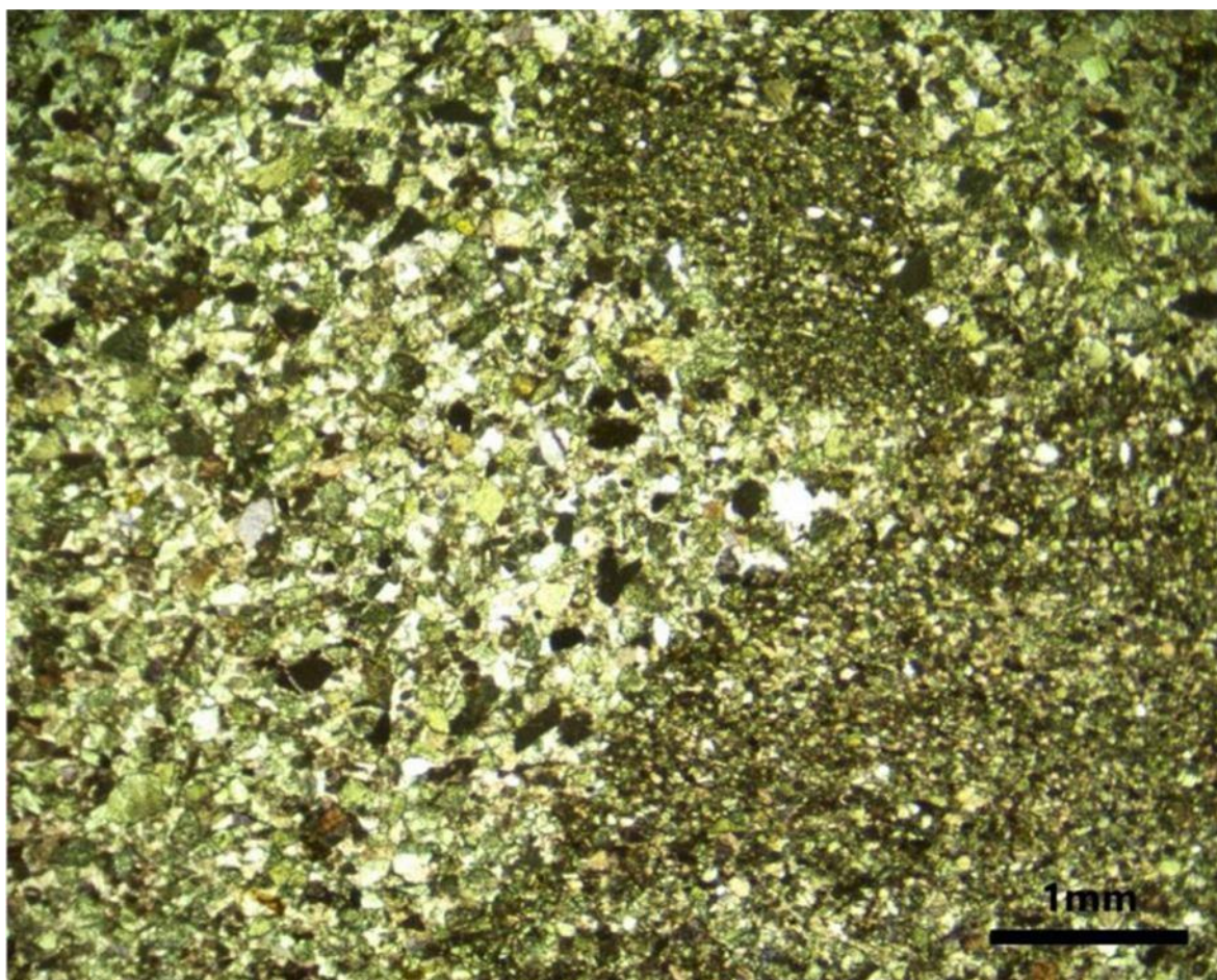
Slika 5-16. Mikropetrološka fotografija pješčenjaka koji izgrađuje Šujičko oligo-miocenski bazen. Pješčenjaci su pretežito izgrađeni od karbonatnih čestica, uz jako malo kvarcnih čestica. Na fotografiji se uočava jasna granica gdje dolazi do izmjene sitnozrnatijeg i krupnozrnatijeg pješčenjaka. Točka istraživanja A 33, koordinate X: 6436538 Y: 4851010.
