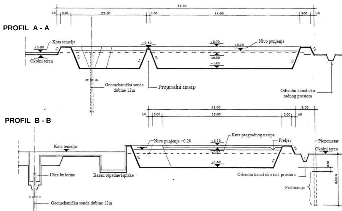
Slika 4-6. Presjeci isplachne jame s položajem piezometara i sonde (Rukavina et al., 1990)
