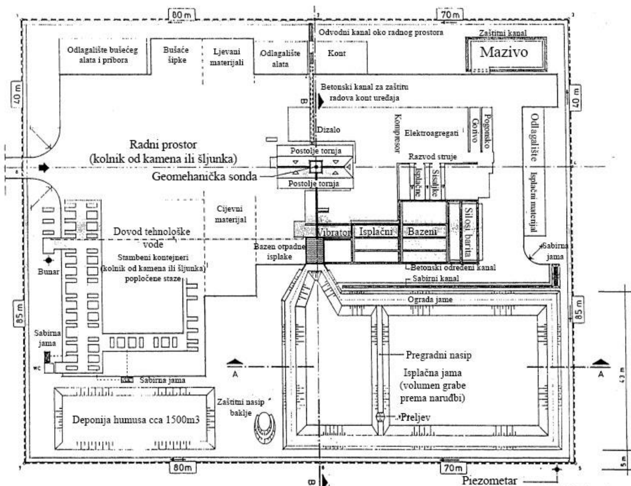
Slika 4-5. Shematski prikaz položaja isplachne jame na prostoru bušotine prema Glavnom tipskom rudarskom projektu (Rukavina et al., 1990)
