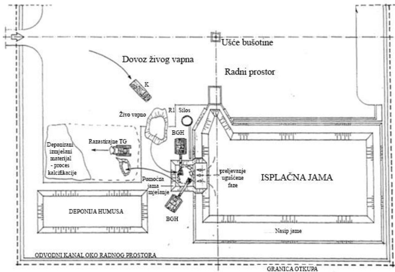
Slika 4-8. Shematski prikaz postupka solidifikacije ugušćene faze građevinskim strojevima – miješanje ugušćene faze u pomoćnoj jami (Rukavina et al., 1990)
