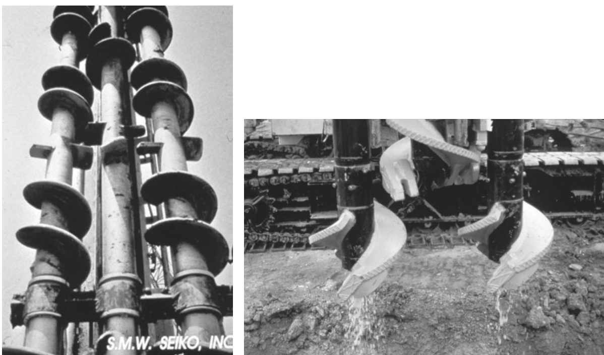
Slika 3-12. Sustav mješača (augera) (Al-Tabbaa i Perera, 2006)
