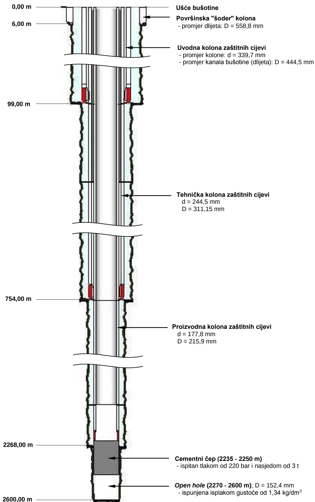
Slika 4-4. Konstrukcija bušotine Hrastilnica-4 (Biletić, 2014)
