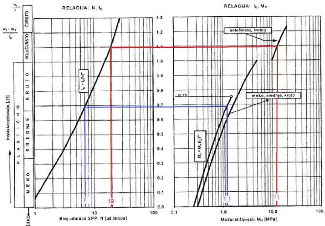
Slika 4-2. Rezultati SPP-a za lokaciju radnog prostora bušotine Hra-4: ispitivanja na površini terena (crvena linija) i na dubini od 80 cm (plava linija) (Milčić et al., 2014)
