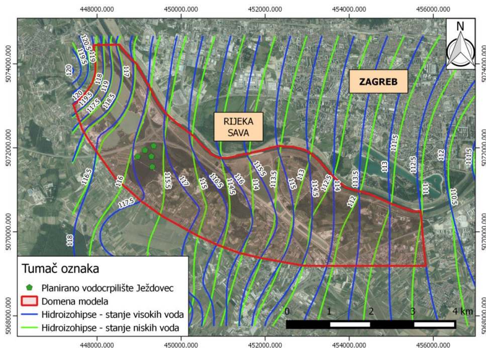
Slika 5.3 Domena modela
