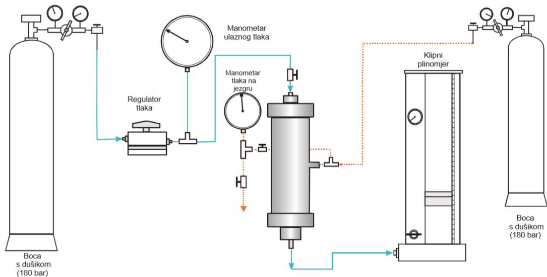
Slika 4-38. Shematski prikaz uređaja za mjerenje propusnosti protokom plina (Vulin, 2012).
