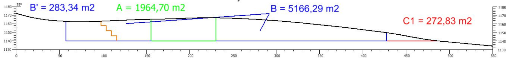
Presjek 7-7'
