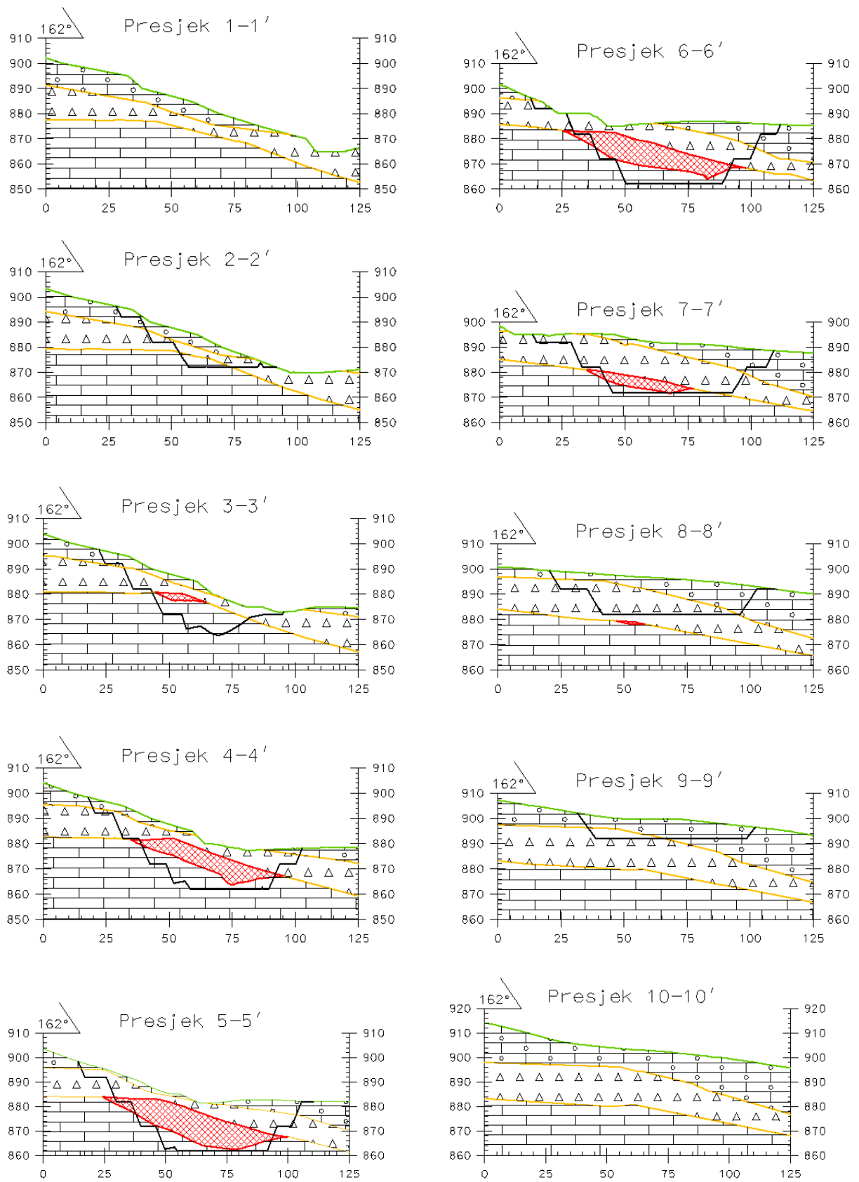
Slika 6-23. Presjeci većeg površinskog kopa, M1:2000
