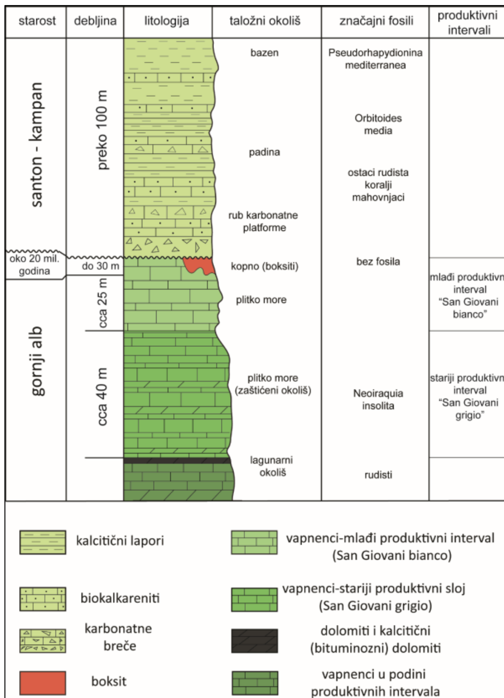
Slika 4-10. Shematski litostratigrafski stup područja Poljane (Dragičević i dr., 2016)
