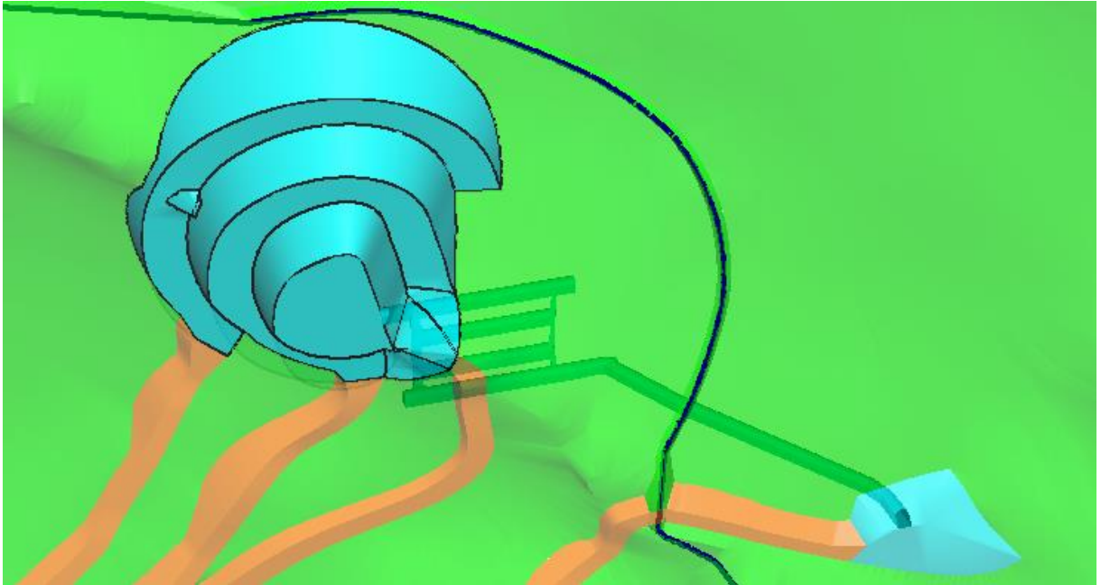
Slika 6-26. Renderirani prikaz manjeg kopa i podzemnih prostorija za eksploataciju ležišta
