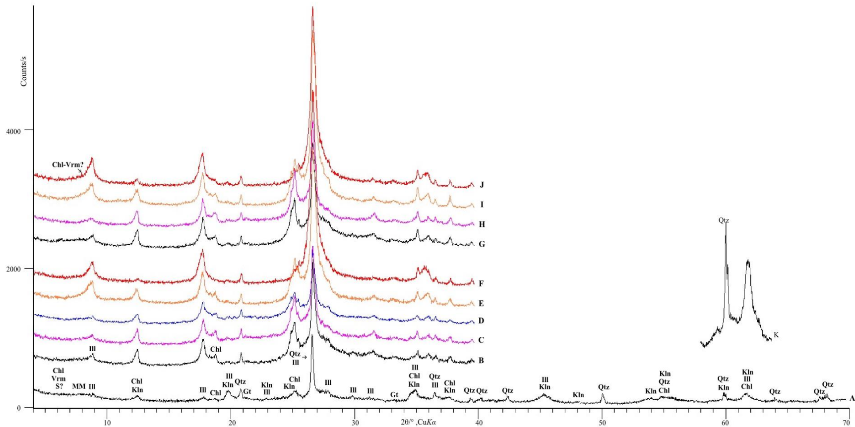
Slika 5-30. Difrakcijske slike glinovite frakcije uzorka 4895 ( A i K predstavljaju snimke neorijetiranih uzorka, a B – J snimke orijetiranih uzoraka): A - netretirani uzorak, B - uzorak tretiran s K^+ , C - uzorak tretiran s K^+ saturiran s etilen-glikolom, D - uzorak tretiran s K^+ saturiran s dimetilsulfoksidom, E - uzorak tretiran s K^+ žaren na 350^\circ C , F - uzorak tretiran s K^+ žaren na 550^\circ C , G - uzorak tretiran s Mg^{2+} , H - uzorak tretiran s Mg^{2+} saturiran s etilen-glikolom, I - uzorak tretiran s Mg^{2+} žaren na 350^\circ C , J - uzorak tretiran s Mg^{2+} žaren na 550^\circ C ; K - difrakcijska linija 060. Tumač kratica: Qtz – kvarc, Chl – klorit, Ill – illitični materijal, Gt – getit, Kln – kaolinit, MM-miješanoslojni minerali glina, Vrm – vermikulit, S – smektit.
