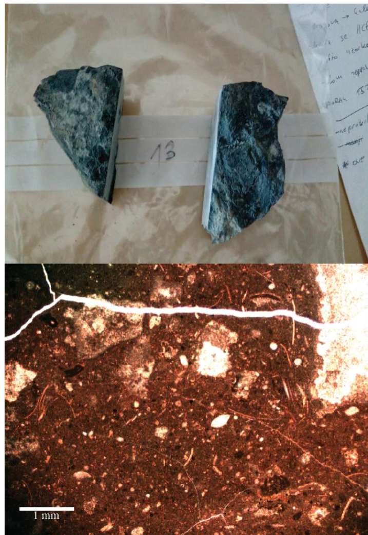
Slika 6.7. Uzorak iz sloja 13 makroskopski uzorak (gore), te veliki broj raznih alokema u mikroskopskom preparatu (dolje).
