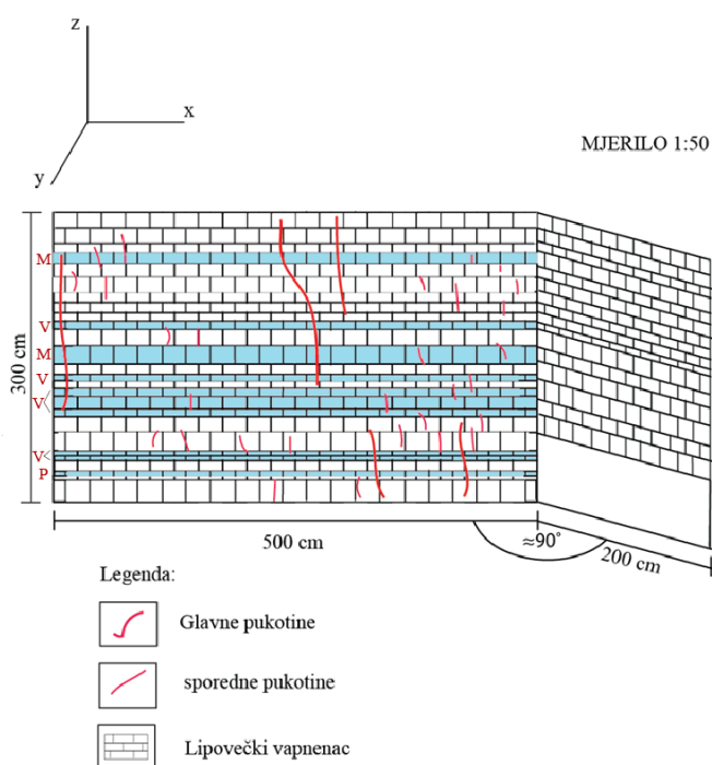
Slika 7.1. Otkopna fronta sa oznakama slojeva i njihovih imena (M - madston, V - vekston i P - pekston).
