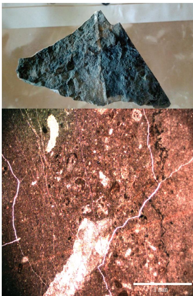
Slika 6.3. Uzorak iz sloja 6 sa vidljivom žilom ispunjenom kalcitom (gore) i tragovi bioturbacija, intraklasta i stilolitski šav (dolje).
