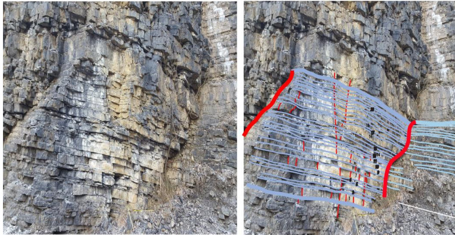
7.5a. Otkopna fronta
