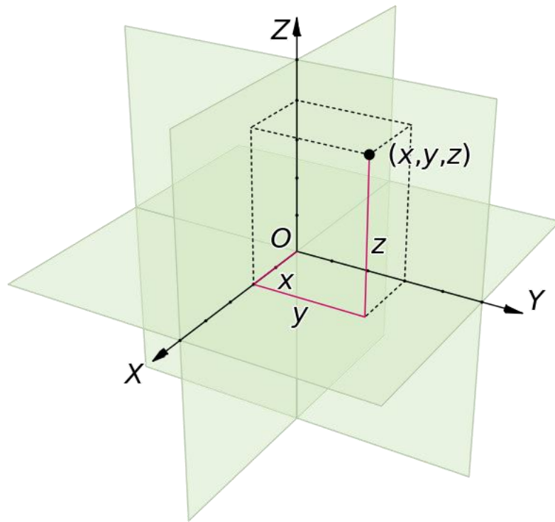
Slika 4.1. Kartezijev koordinatni sustav
