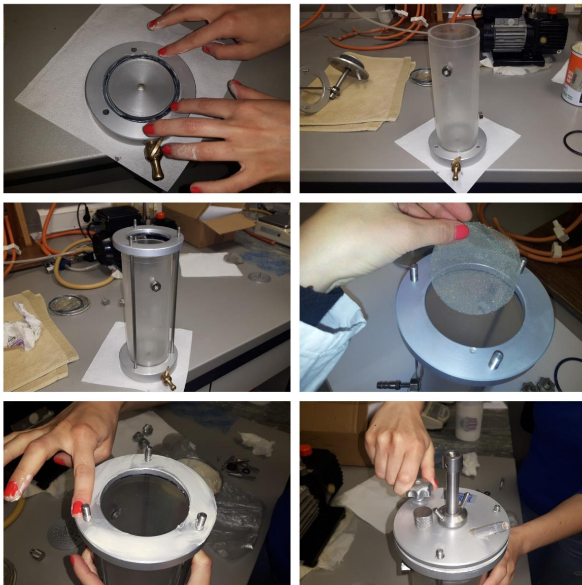
Slika 4-10 Sastavljanje ćelije
