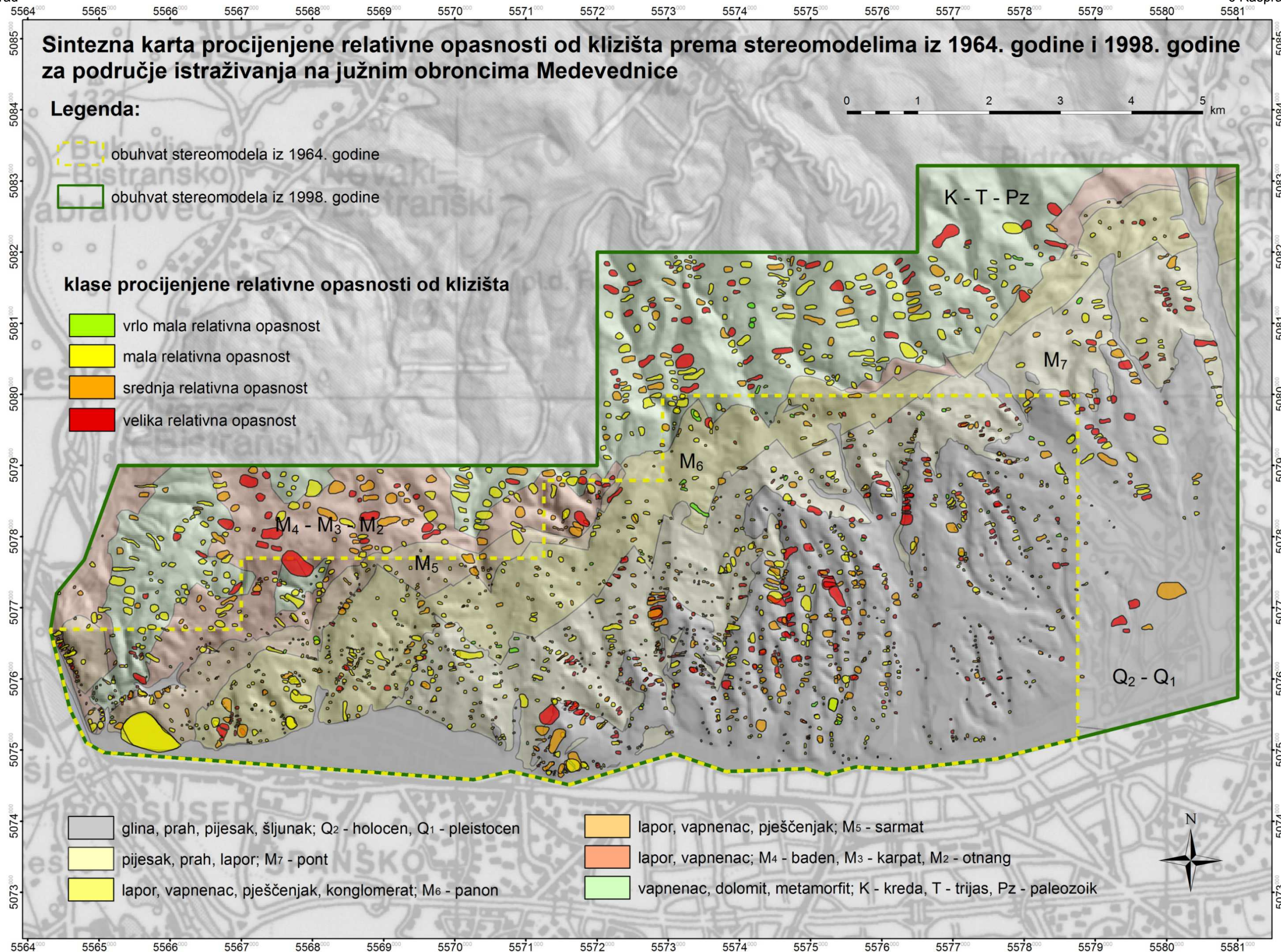
Slika 108 Sinteza karta procijenjene relativne opasnosti klizanja prema stereomodelima iz 1964. godine i 1998. godine za područje istraživanja na južnim obroncima Medvednice s prikazom klasifikacije klizišta utvrđenom pomoću AHP metode (detaljno opisano u poglavlju 4.2.2)
