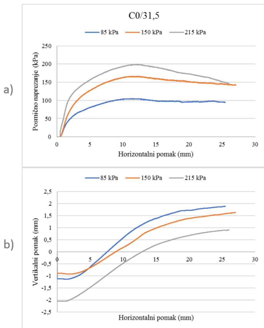
Slika 4-8 Dijagrami a) Horizontalnog pomaka i posmičnog napreznja i b) Horizontalnog pomaka i vertikalnog pomaka za frakciju C0/31,5
