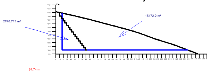
Presjek 3-3'
