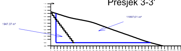
Presjek 3-3'
