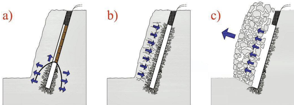
Slika 2-1. Djelovanje detonacije eksploziva u minskoj bušotini (Škrlec et al., 2014)
