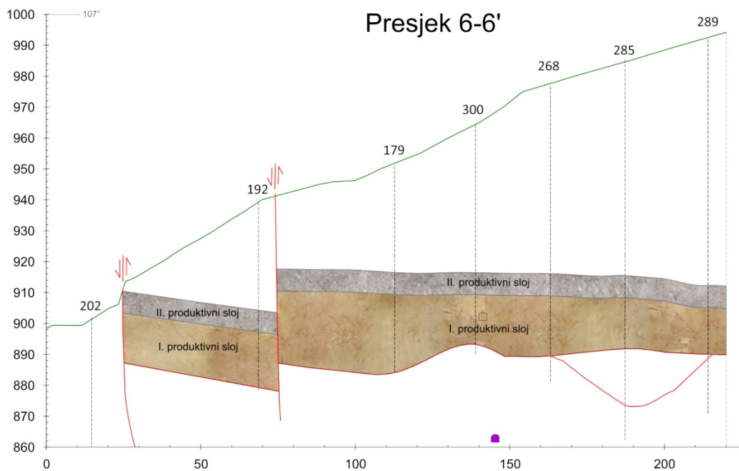
Slika 27 – Pripremljeni obračunski presjek 6 – 6' s iscrtanim ploham produktivnih slojeva
