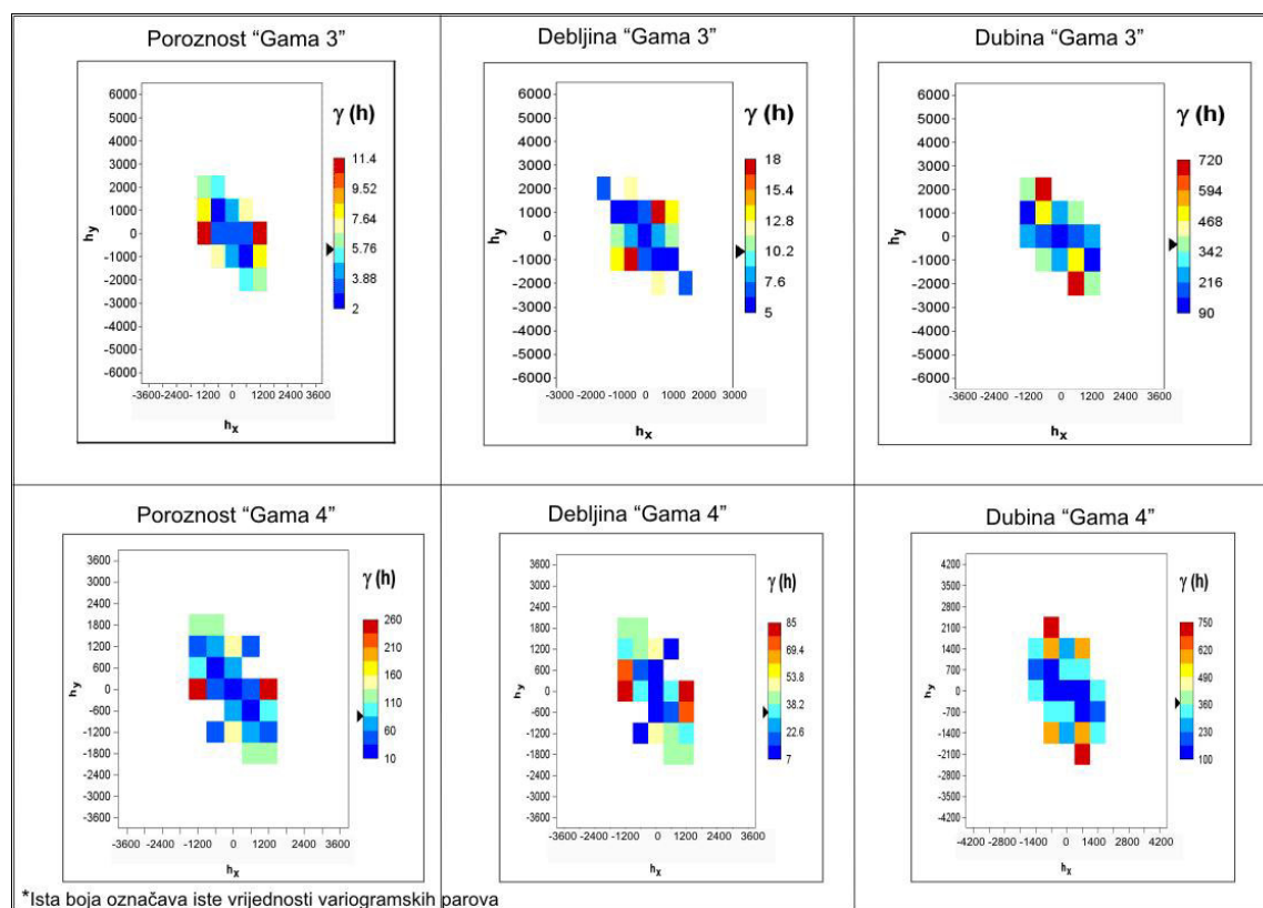
Slika 6-1. Karte variogramskih površina za varijable poroznost, debljinu i dubinu ležišta Gama 3 i Gama 4
