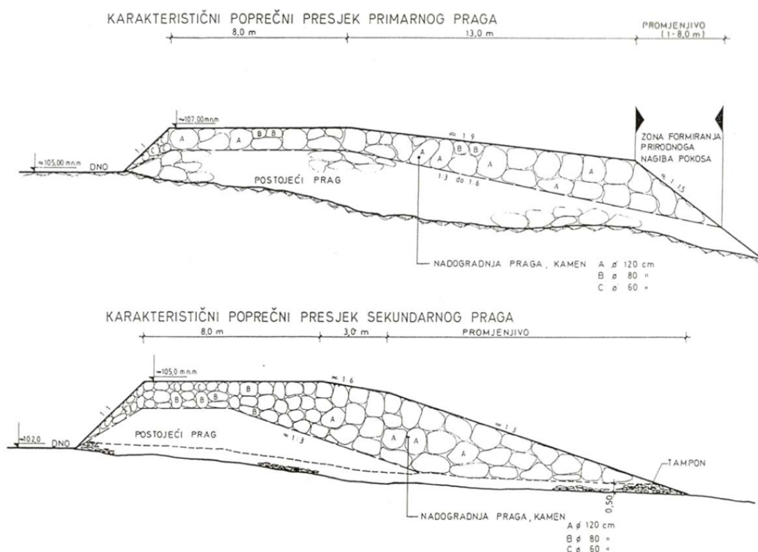
Slika 2.5. Karakteristični poprečni presjeci nadograđenog primarnog i sekundarnog praga te njihovo stanje prije nadogradnje (preuzeto iz Biondić, 1995)
