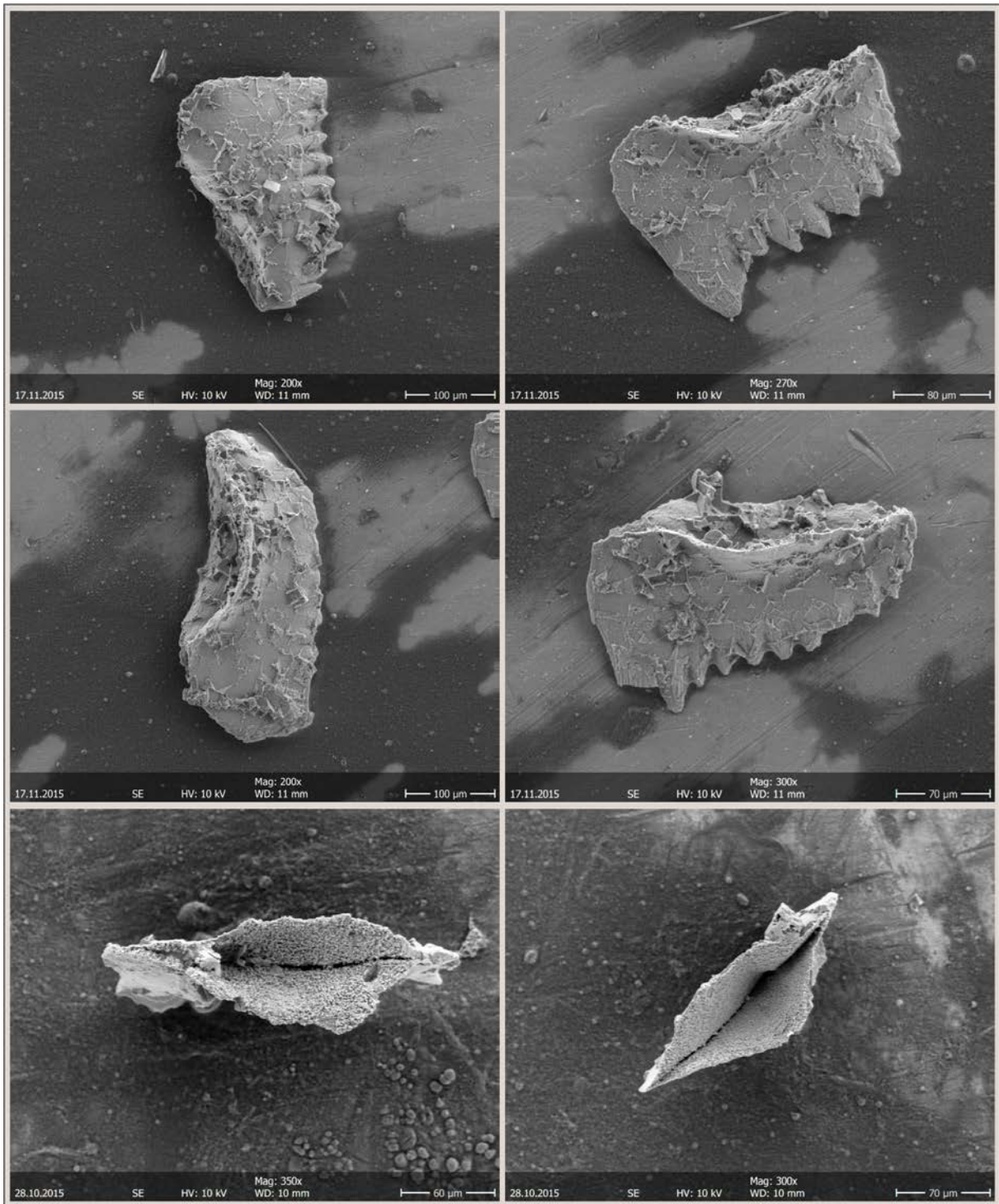
Slika 7.8: SEM fotografije konodontata prikupljenih iz slojeva Sy37 i Sy38 slijeda Brušane Sy (fotografije ustupio Dr. sc. Yanlong Chen)
