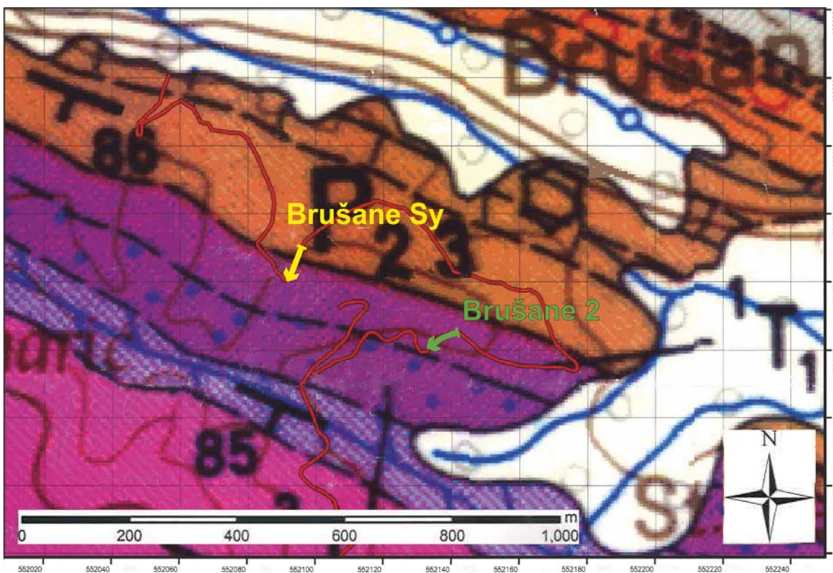
Slika 5.1: Geološka karta istraživanog područja (isječak iz Osnovne geološke karte mjerila 1:100 000 list Gospić-104, SOKAČ et al., 1967a) s označenim profilima Brušane Sy (žuto) i Brušane 2 (zeleno). Crvena linija predstavlja šumsku cestu.
