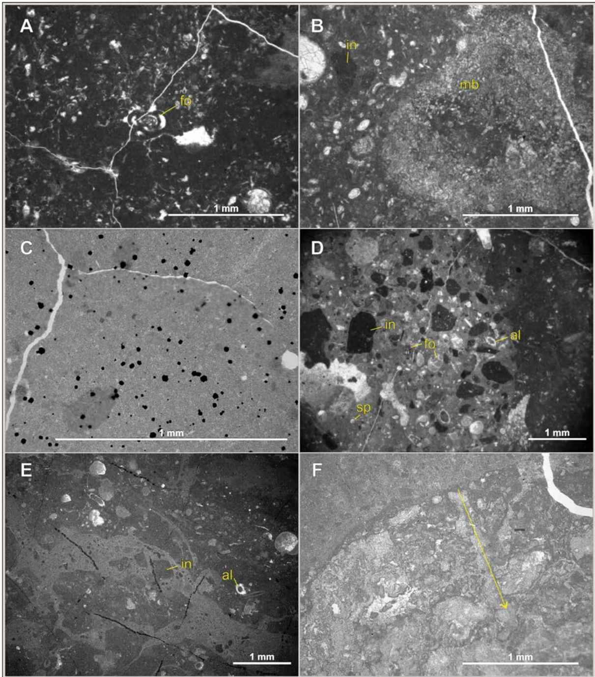
Slika 7.4: Mikrofotografije uzoraka stijena slijeda Brušane Sy: A – Sy32 (fo – foraminifera; dolomikrit/madston); B – Sy28 (mb – cijanobakterije,; dolobiomikrit/vekston); C – Sy17b (pirit; dolomikrit/madston); D – Sy33 (fo – foraminifera, al – vapnenačka alga, sp – spore algi, in – intraklasti; dolobiomikrit/vekston); E – Sy7 (in – intraklasti, al – vapnenačka alga; dolobiomikrit/vekston); F – Sy11 (žuta strelica – smjer bioturbacije; dolomikrit/madston)
