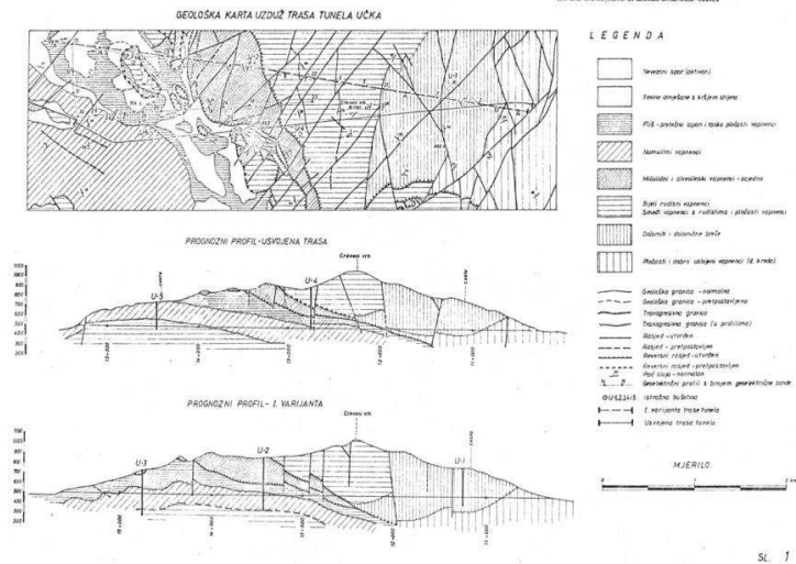
Slika 3-3. Inženjersko-geološka karta s pripadajućim profilima.
