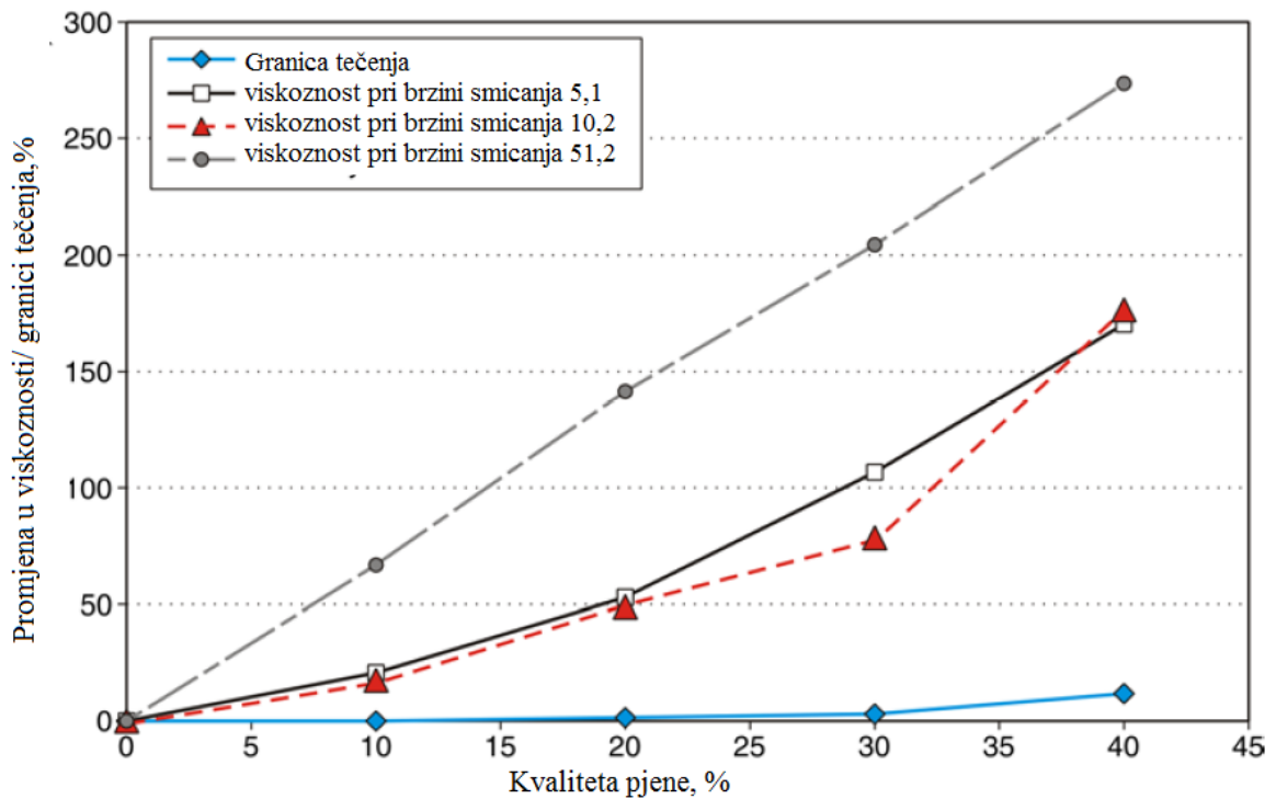
Slika 3-12. Utjecaj kvalitete pjene na promjene naprezanja pri pokretanju i viskoznosti pjenocementne kaše koristeći Fann viskozimetar (Olowolagba i Brenneis, 2010)
