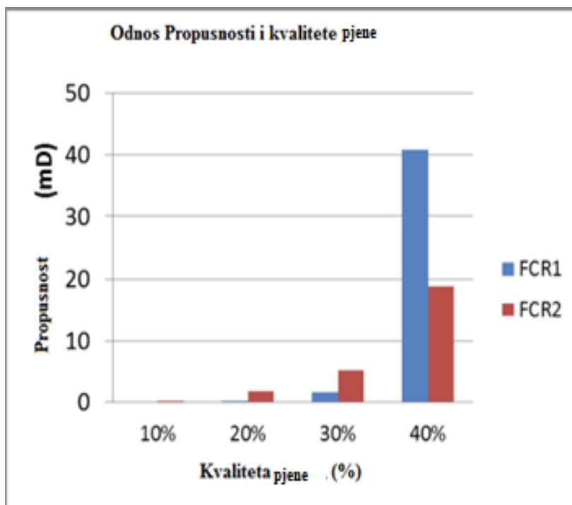
Slika 5-10. Odnos propusnosti i kvalitete pjene za pjenocementnu kašu recepture FRC1 i FRC2 (Kutchko i dr., 2014)
