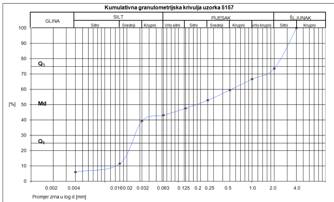
Slika 6-23. Kumulativna granulometrijska krivulja uzorka 5157
