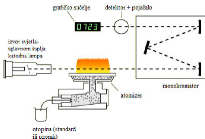
Slika 4. Princip rada atomske apsorpcijske spektrometrije [23]
