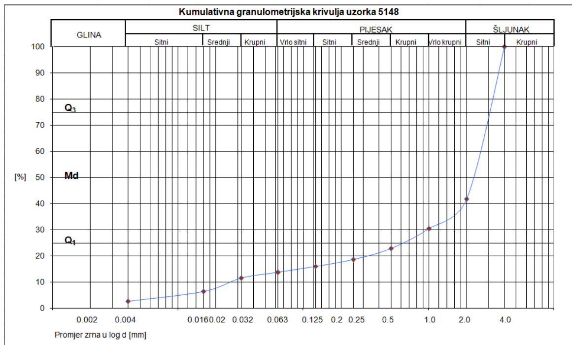
Slika 6-5. Kumulativna granulometrijska krivulja uzorka 5148
