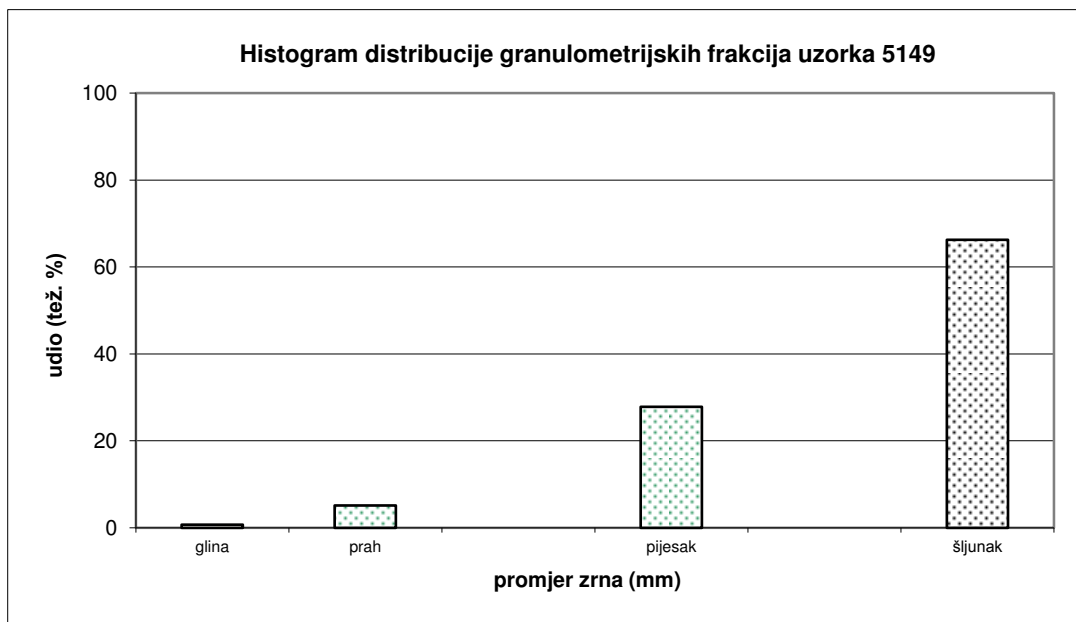
Slika 6-8. Histogram distribucije granulometrijskih frakcija uzorka 5149
