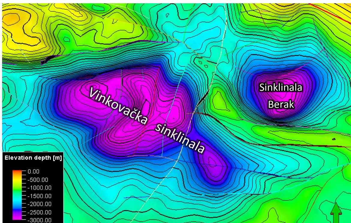
Slika 6-4. Označene su dvije najdublje sinklinalne Slavonko-srijemske depresije.
