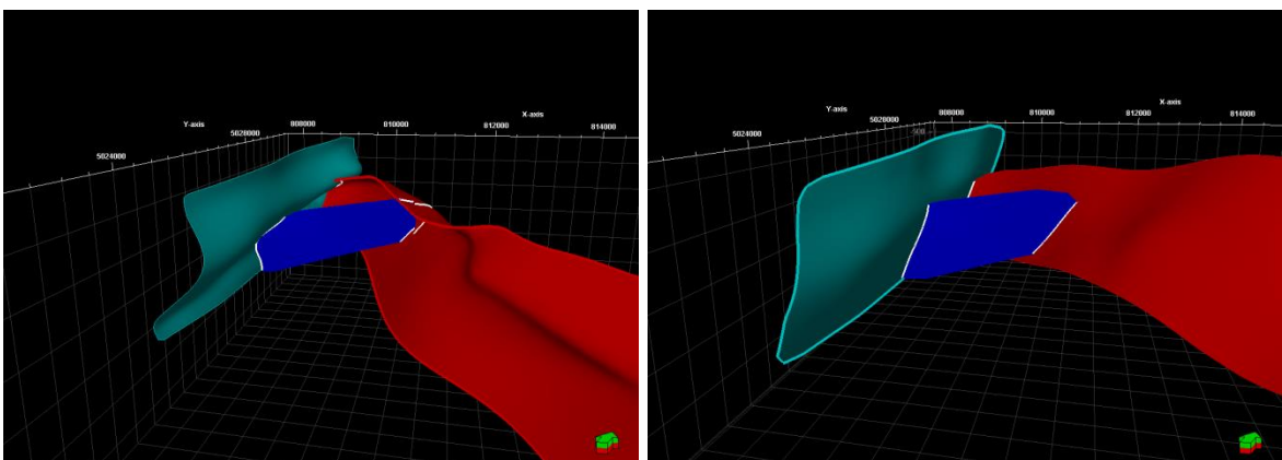
Slika 4-13 (a i b). Lijevo (a) su prikazani pogrešno generirani rasjedi, a desno (b) isti rasjedi nakon ispravljanja.
