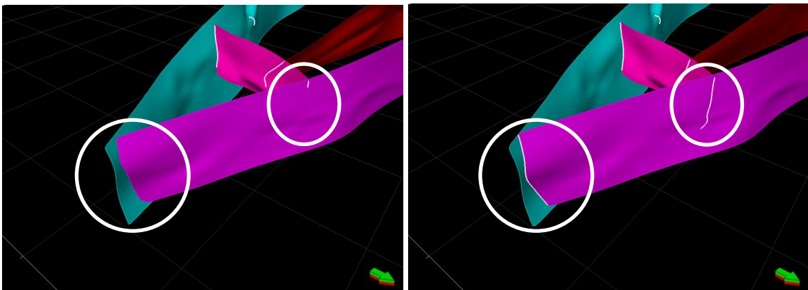
Slika 4-15 (a i b). Primjer popravljivanja kontakta među rasjedima povećanjem udaljenosti ekstrapolacije. Bijela linija na kontaktu znači da je kontakt potpun.
